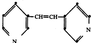
P-20 Trans-1-(3-pyridyl)-2-(4-pyridyl)ethylene:
