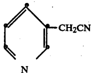
P-20 Trans-1-(3-pyridyl)-2-(4-pyridyl)ethylene:
