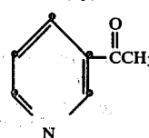
3-Acetylpyridine:
