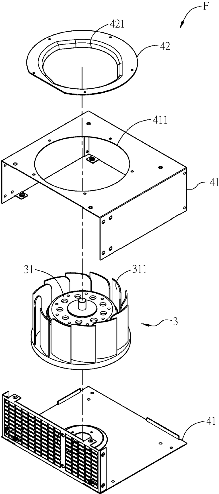
FIG.2B
