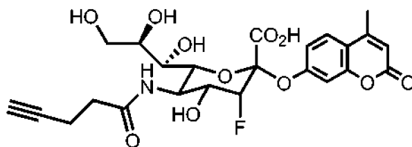
CoumFSA (601)
