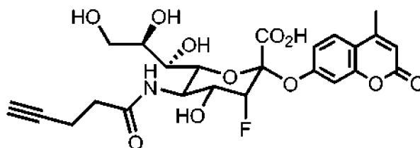
CoumFSA (601)
