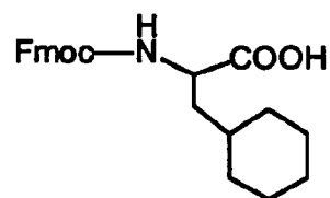
Fmoc-Cha-OH
