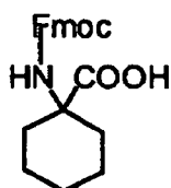
Fmoc-Ac6c-OH
