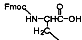
Fmoc-2-Abu-OH
