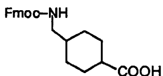
Fmoc-Amc-OH
