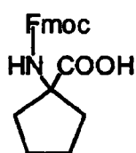
Fmoc-Ac5c-OH
