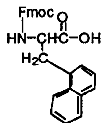
Fmoc-L-1-Nal-OH
