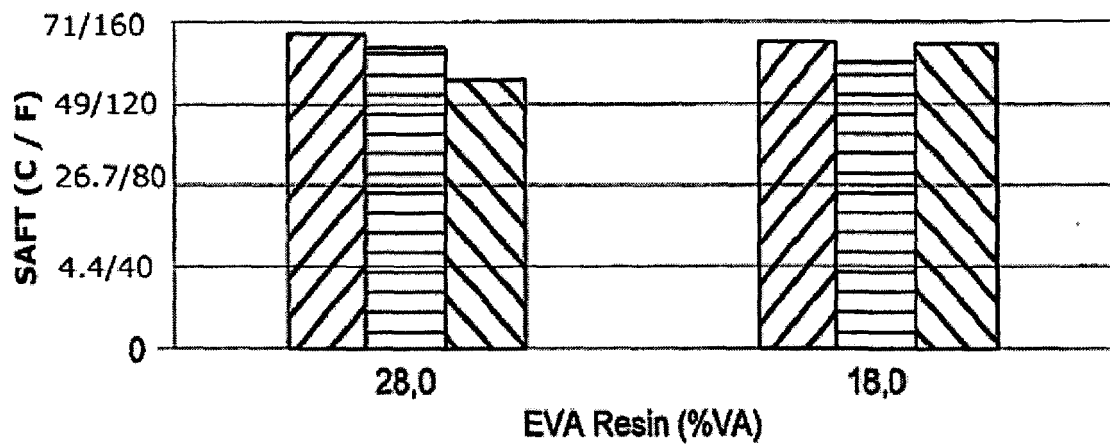
FIG. 4 SAFT (F) ASTM D-4498
