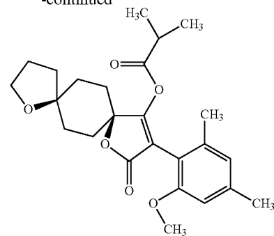
I-2-b-1
