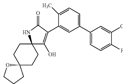
I-1-a-1 20
