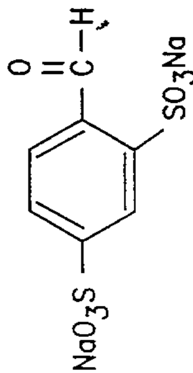
4-Formyl-1,3-benzenesulfonic Acid
