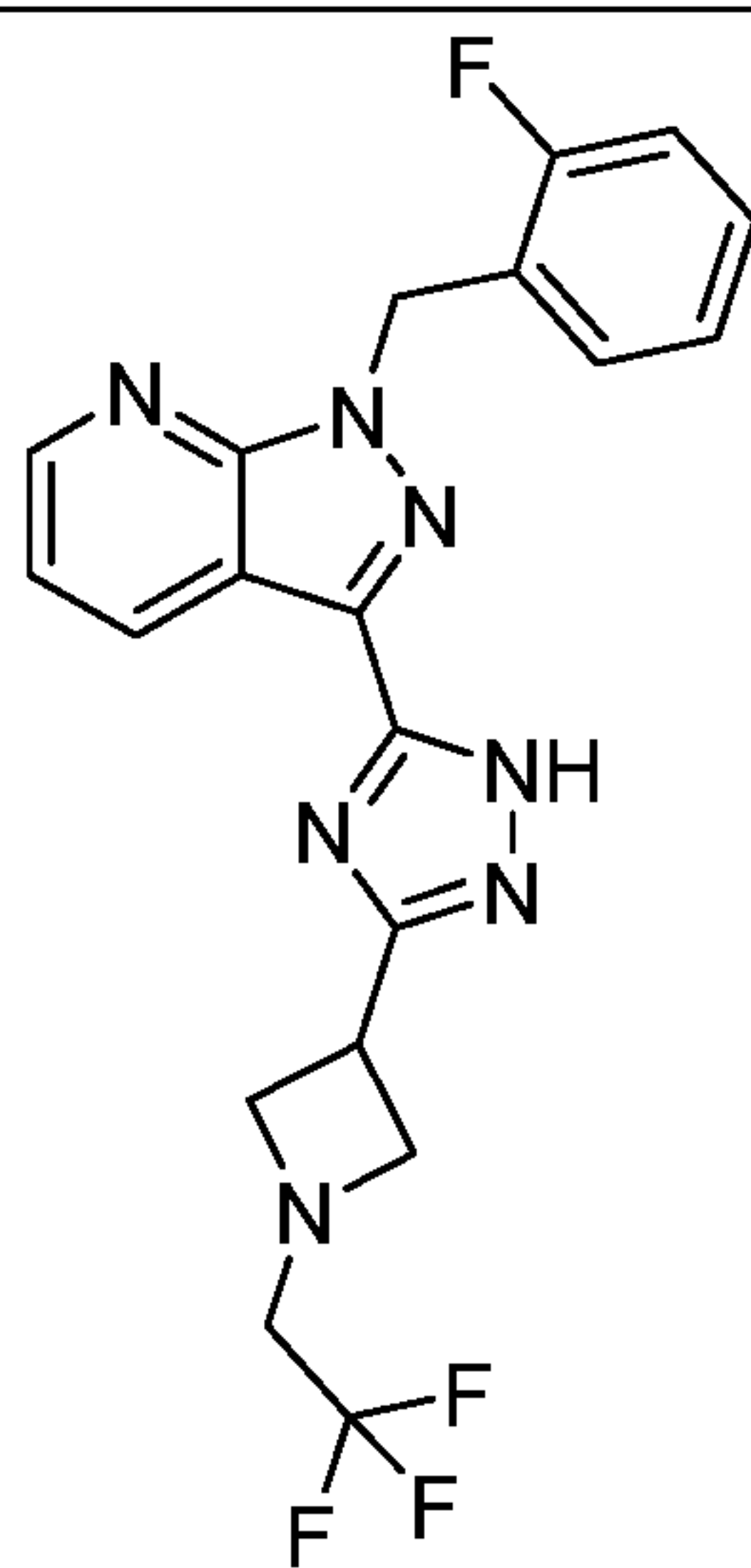
I-95
