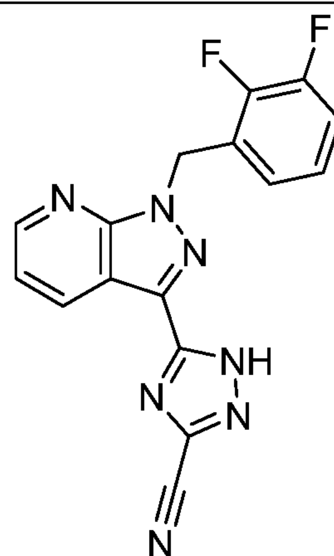
I-92
