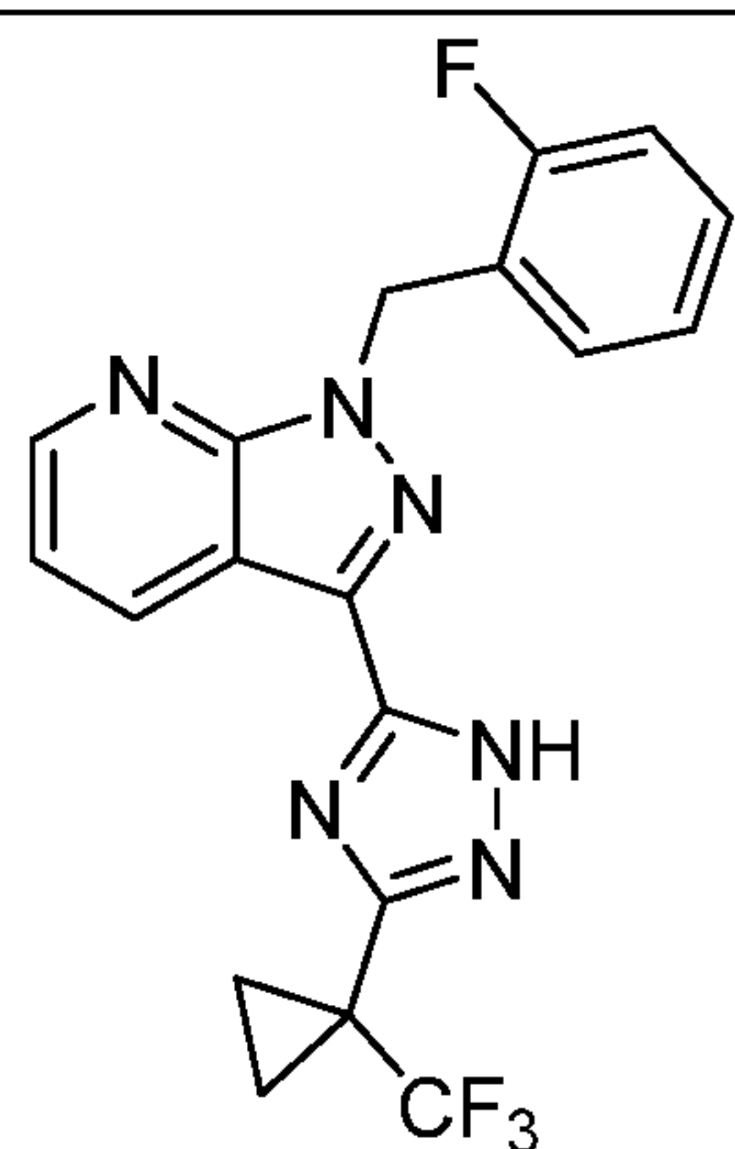
I-59
