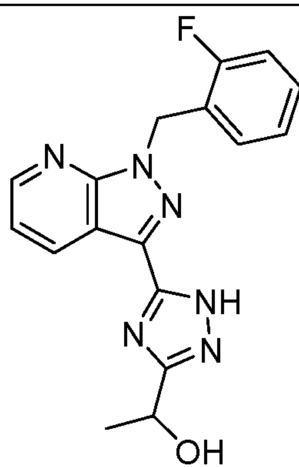
I-107
