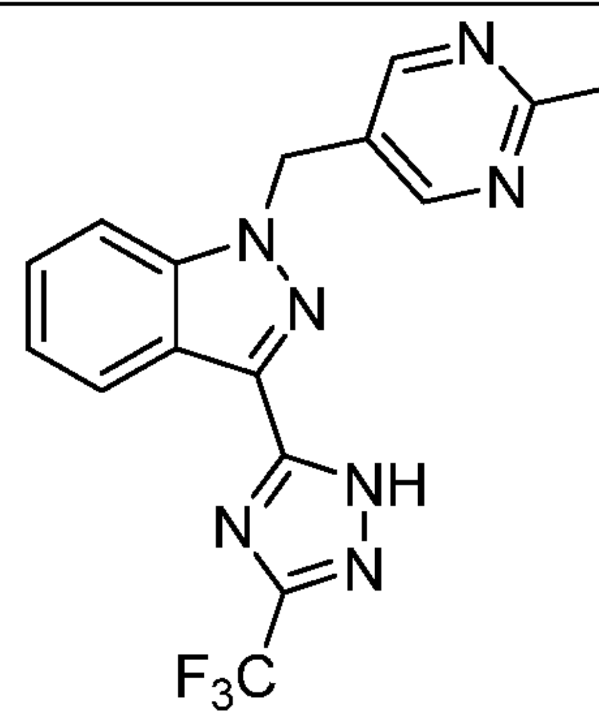
I-62
