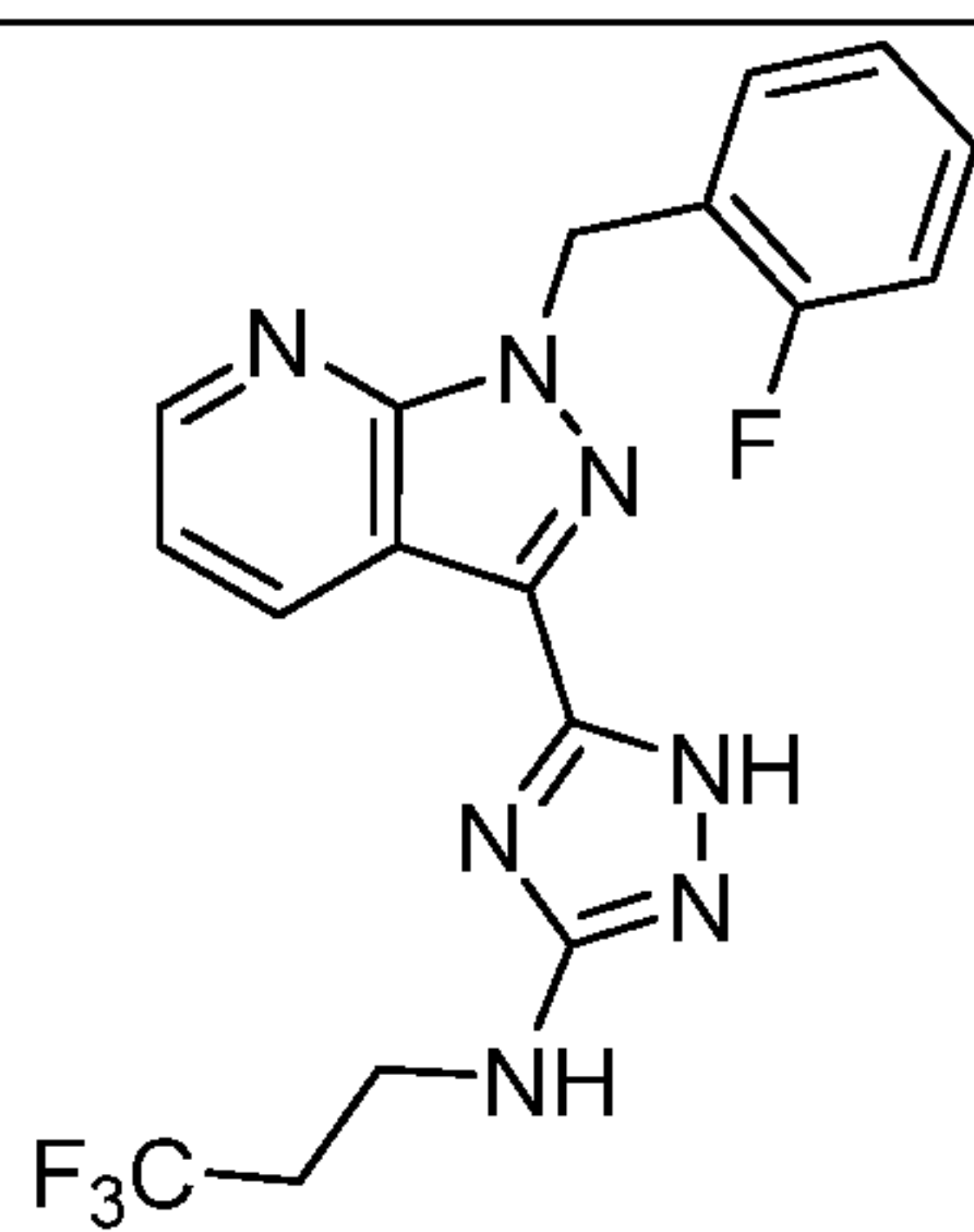
I-89
