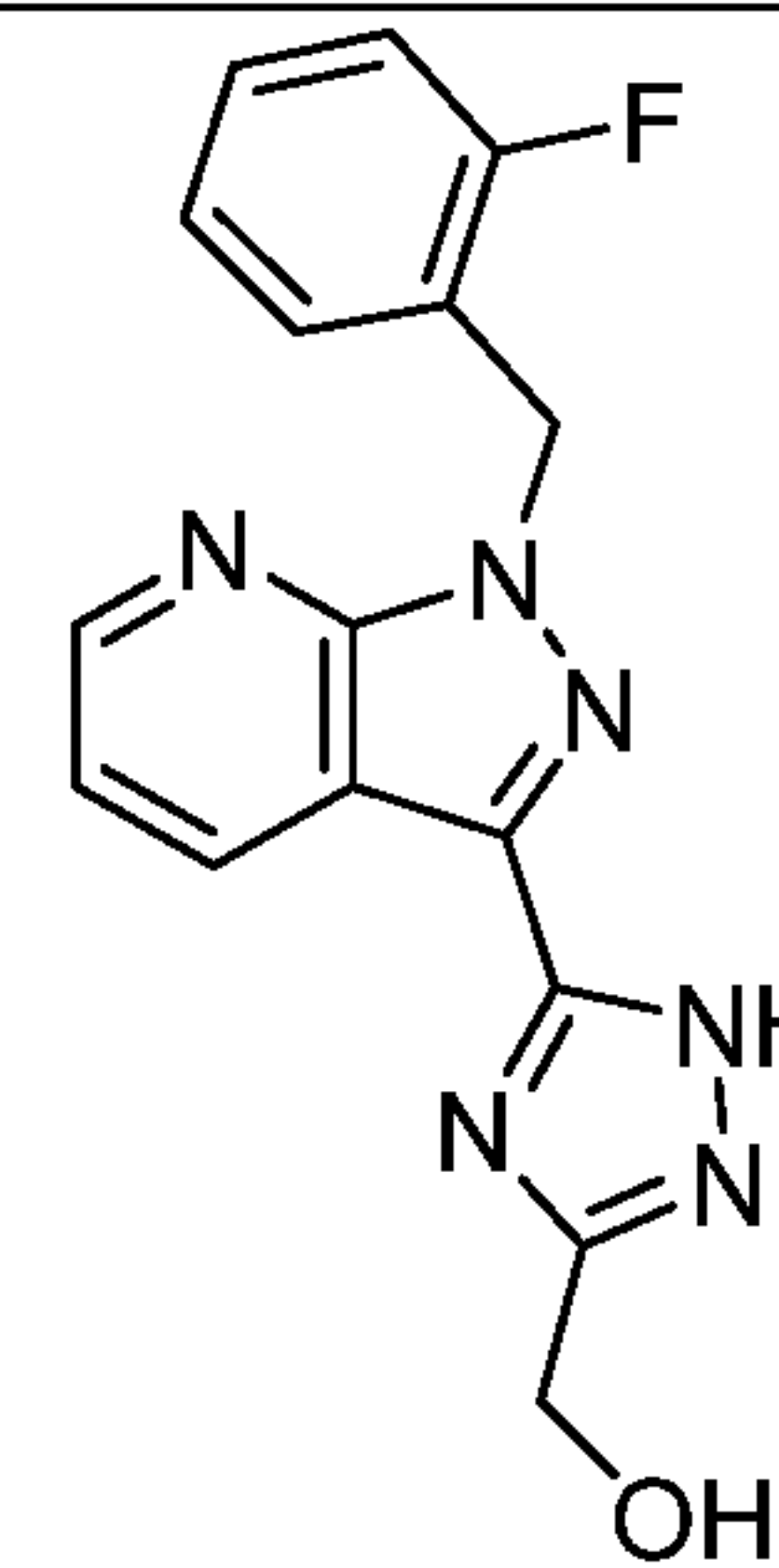
I-64
