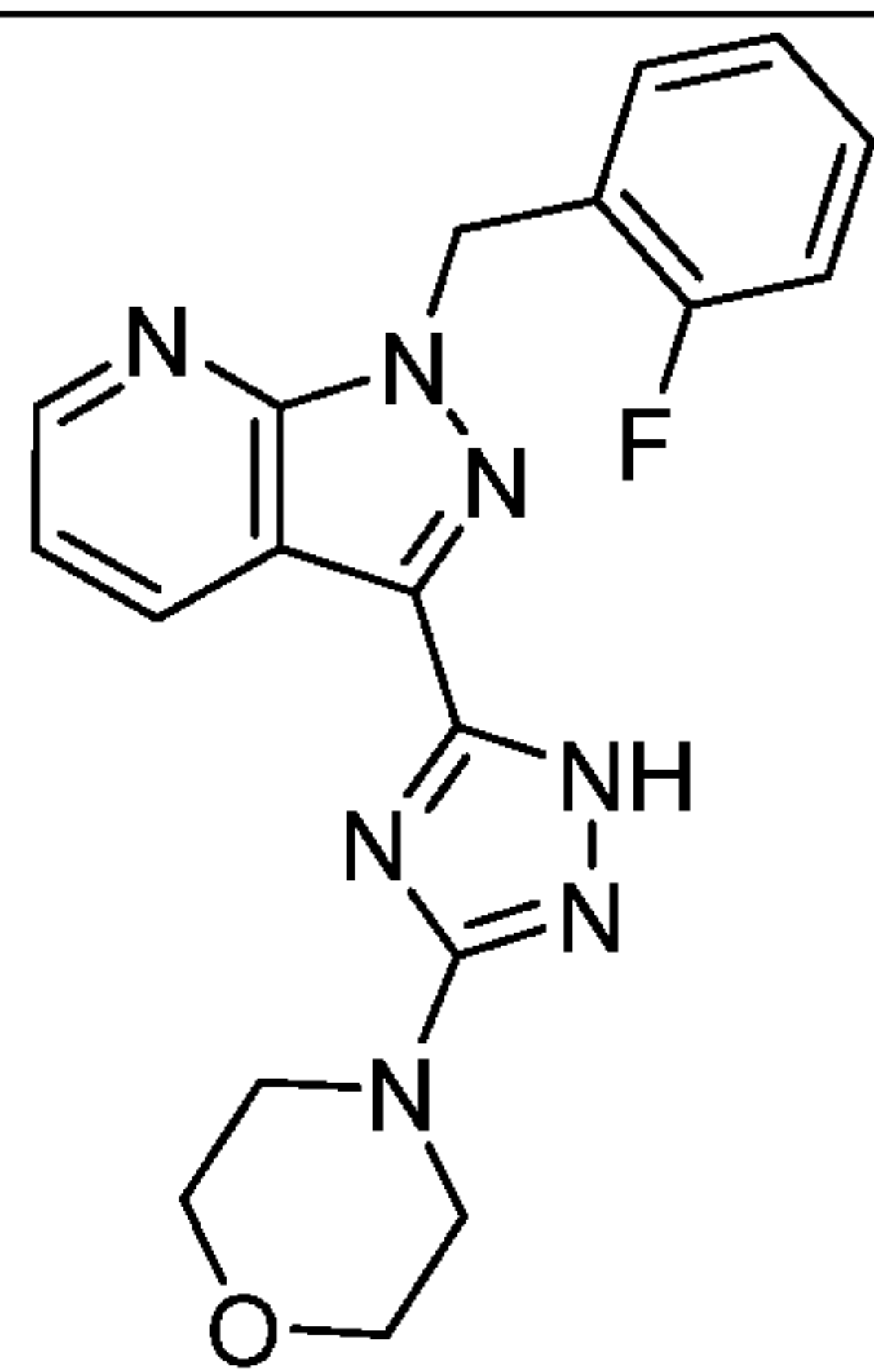
I-57
