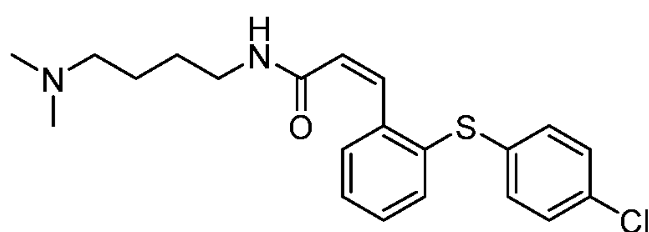
A350619;
