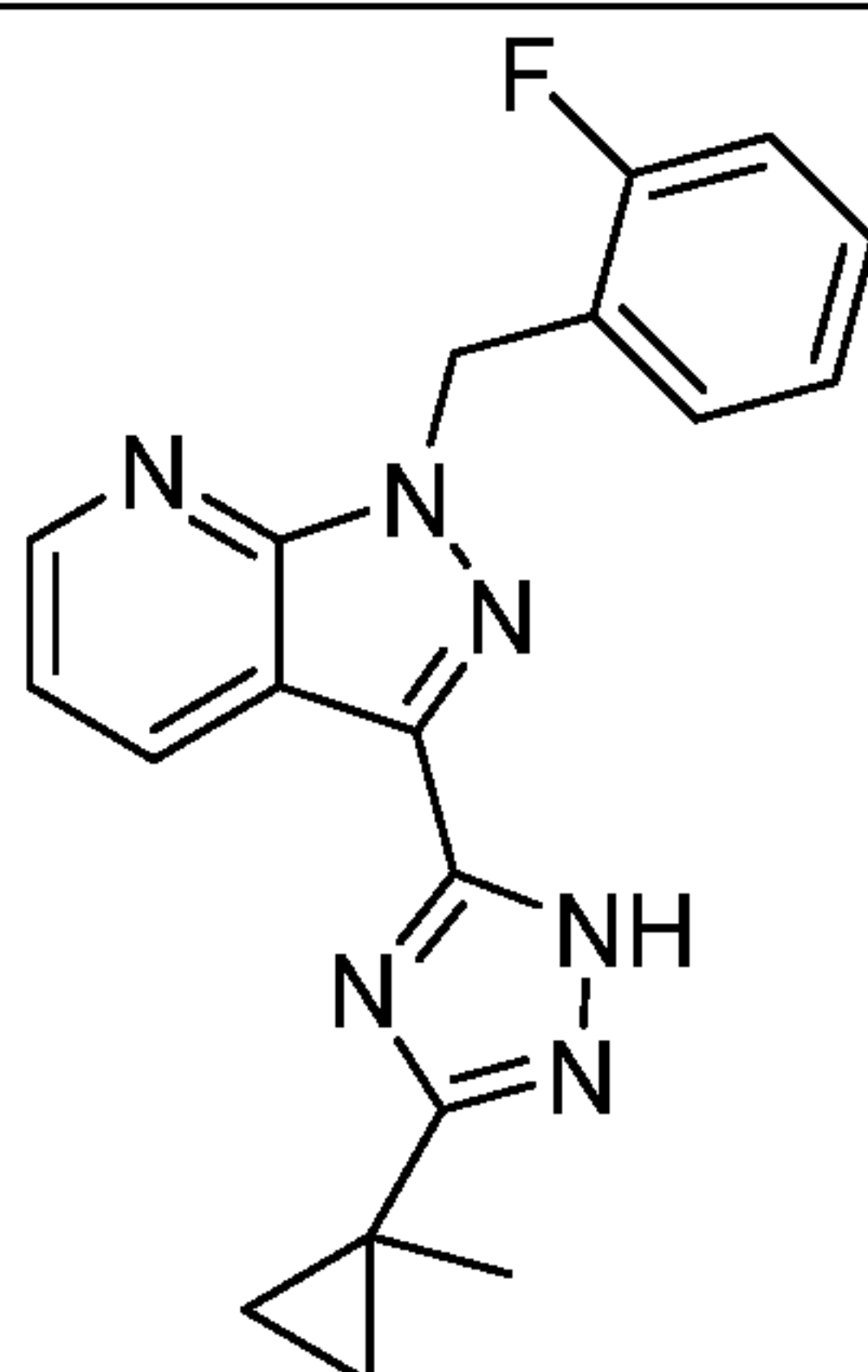
I-63
