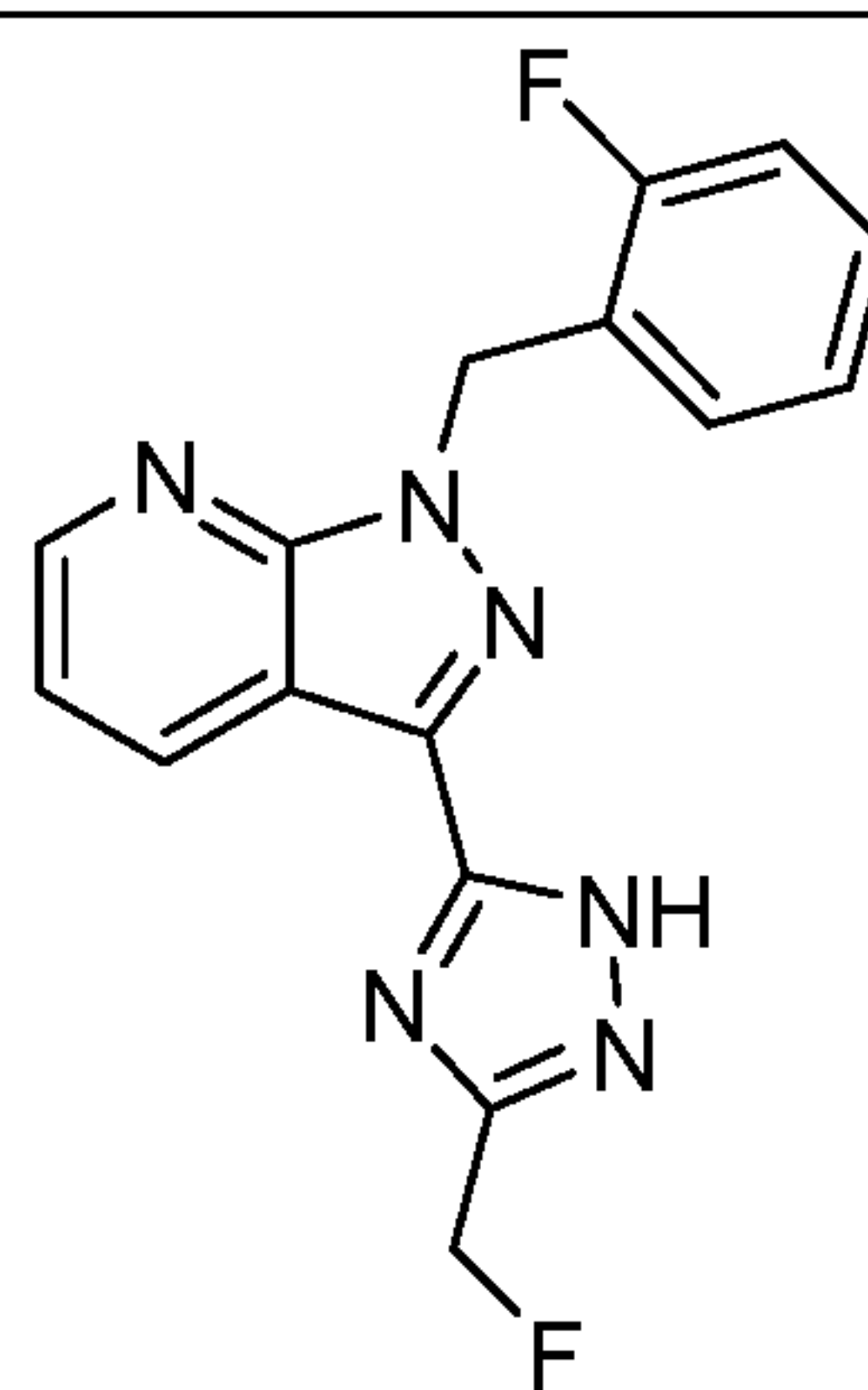
I-58
