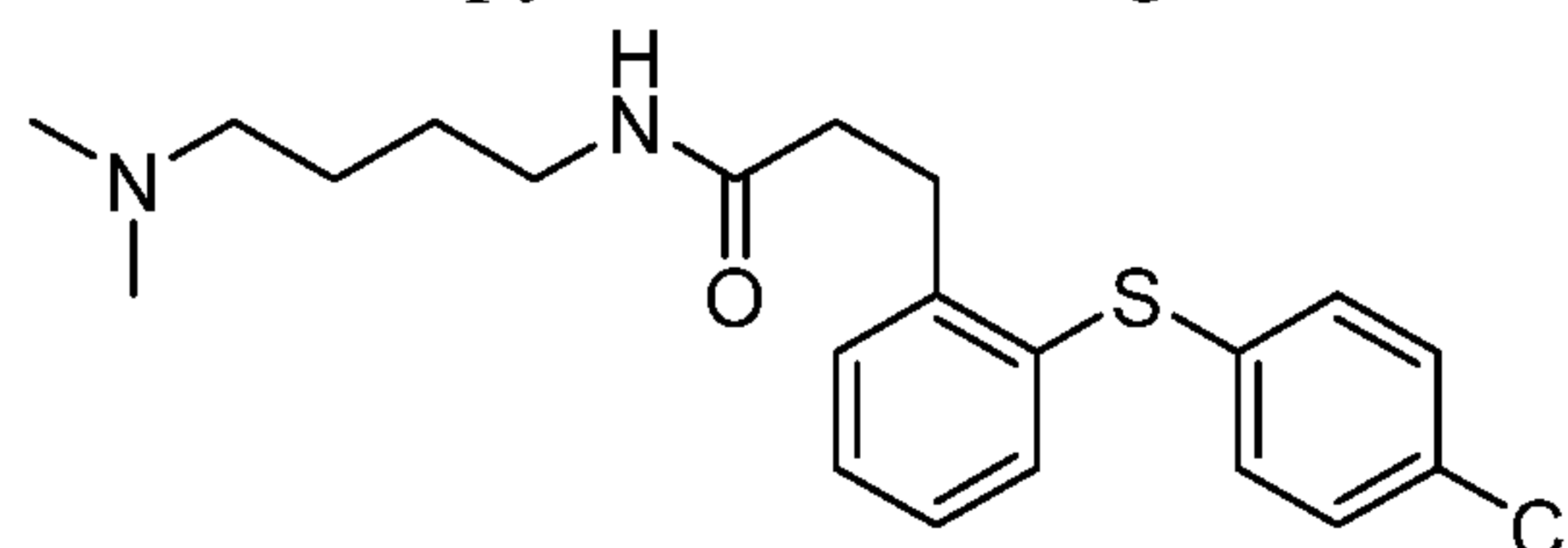
A-344905;
