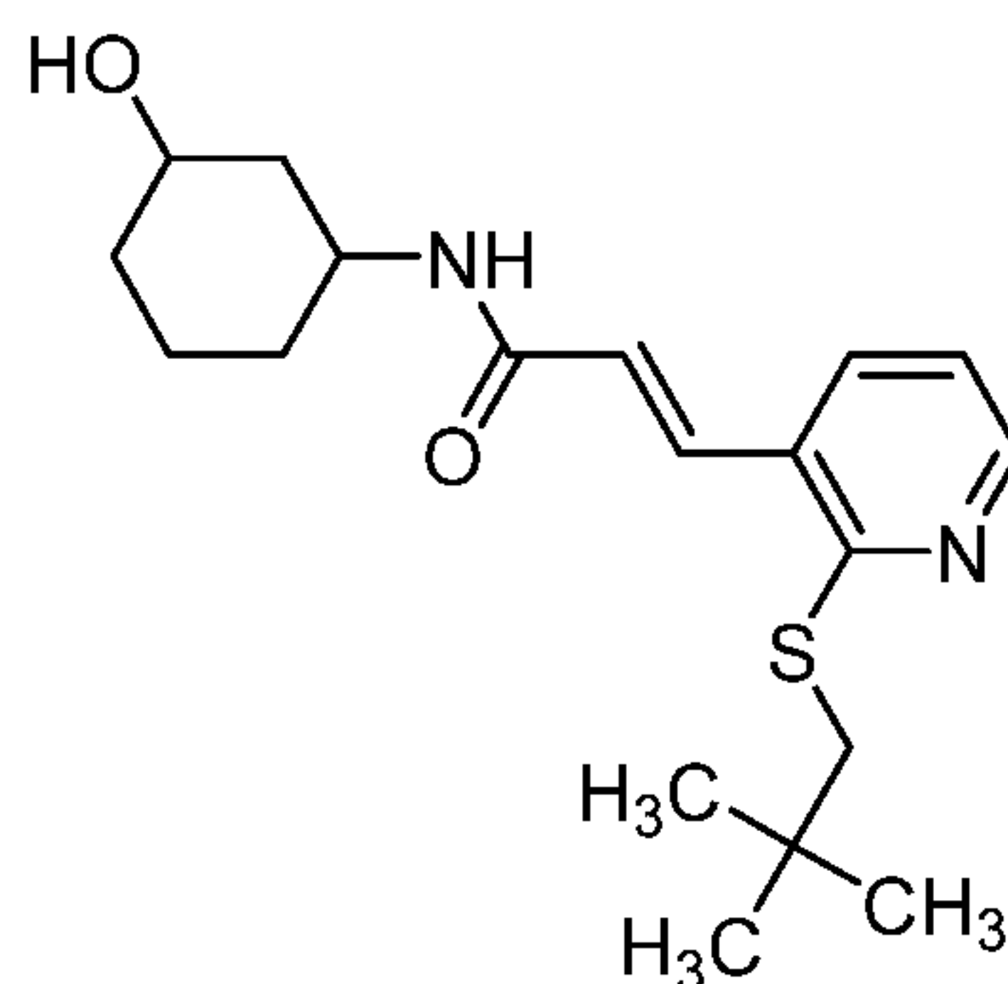
A-778935;
