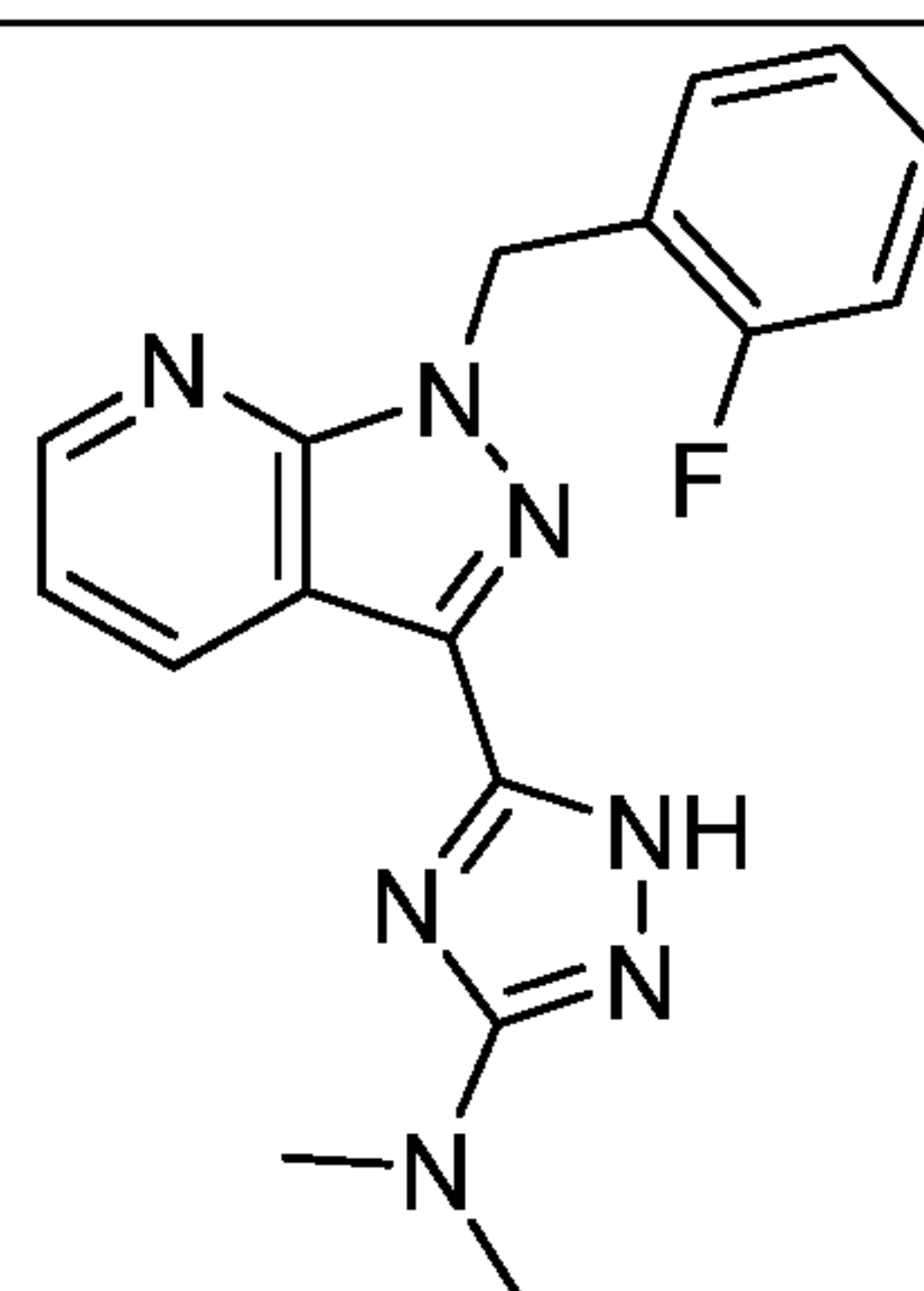
I-90
