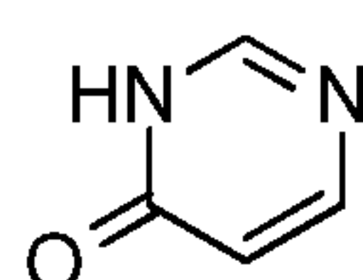
D7
