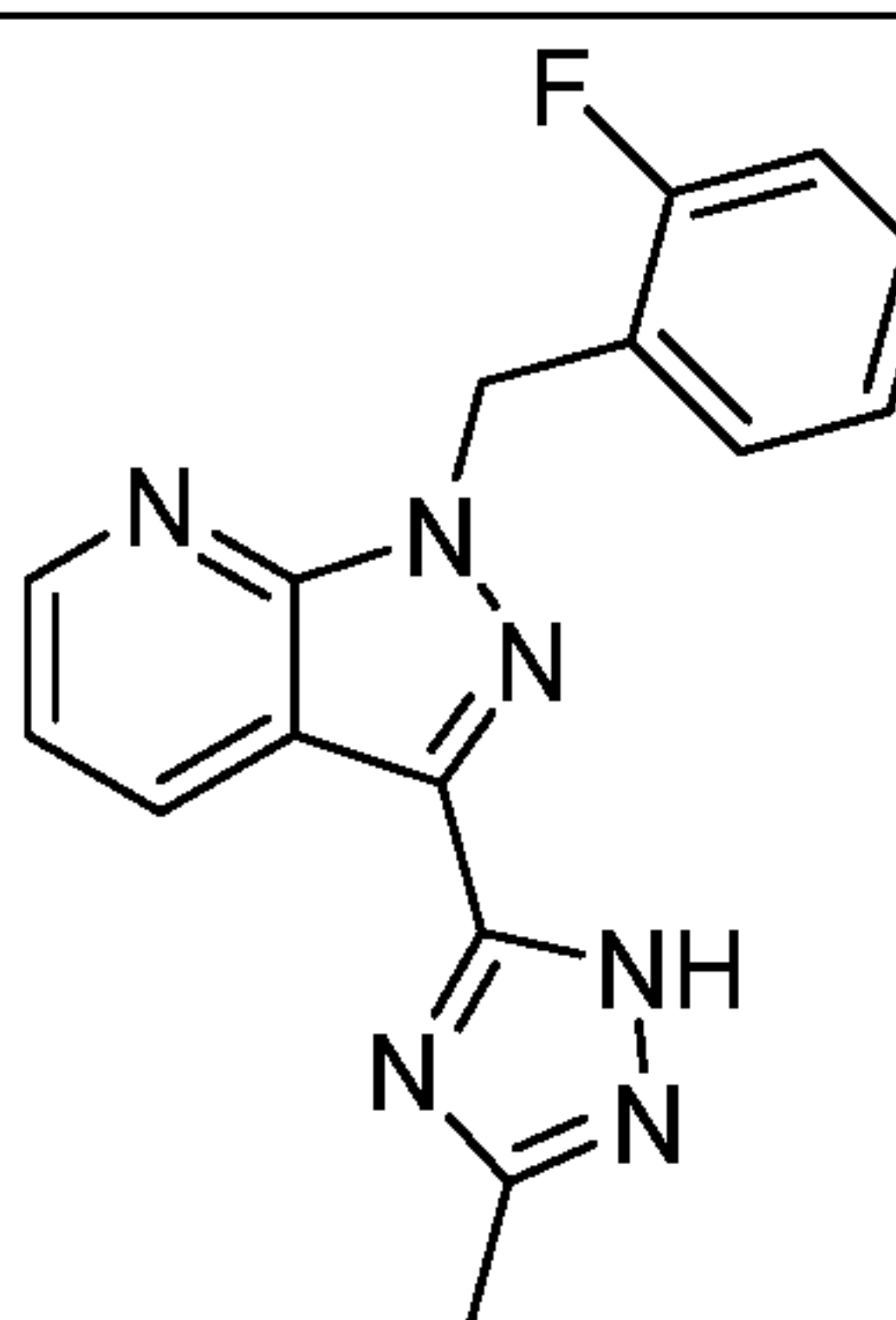
I-60
