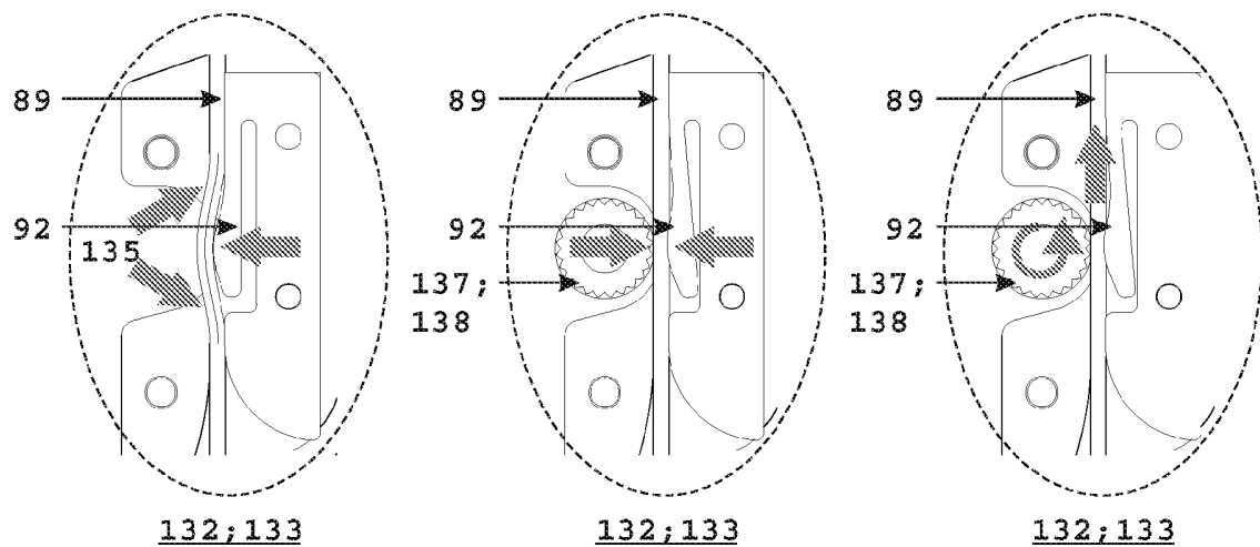
Fig. 17: Federplatte und Vorschubeinheit (ausgekoppelt / eingekoppelt / mit Vorschub)
