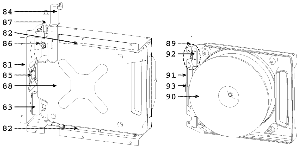
Fig. 16: Versorgungseinheit und Materialkassette (Innenansicht)
