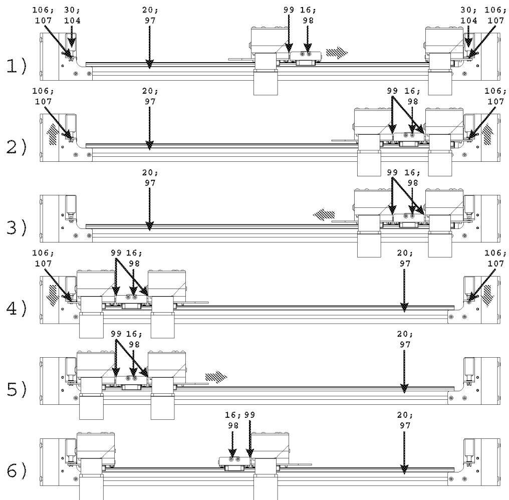
Fig. 7: Automatischer Druckkopfwechsel
