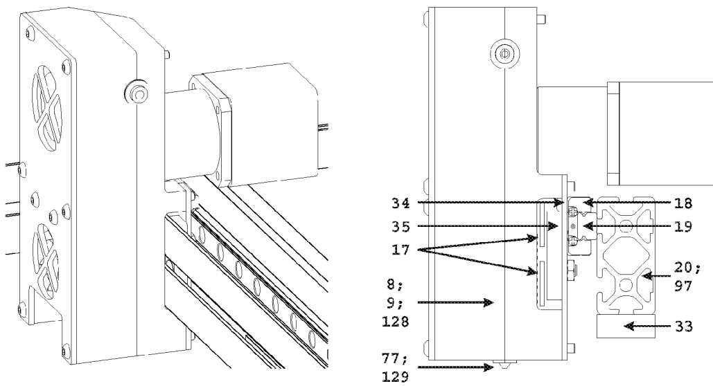
Fig. 6: Druckkopfbefestigung und Führungssystem
