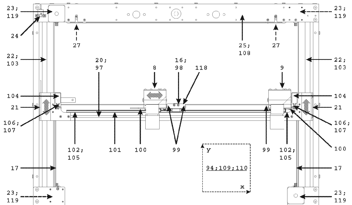
Fig. 3: Horizontales Positioniersystem (Blick von oben)
