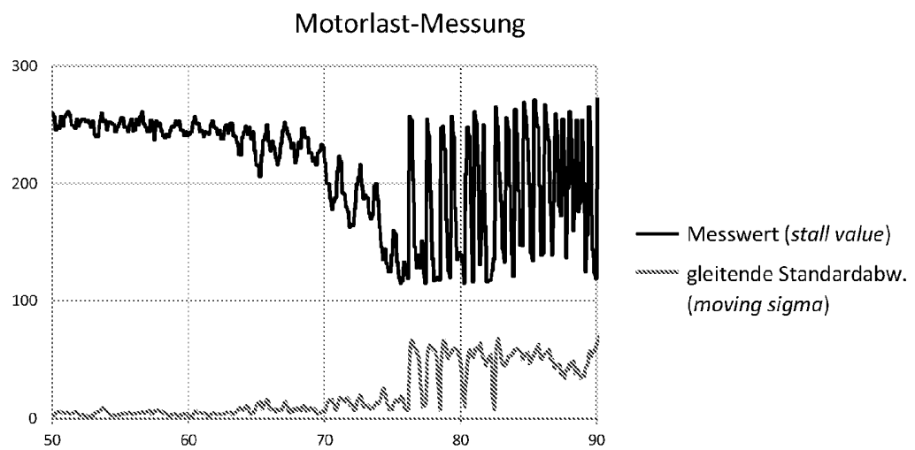
Fig. 15: Motorlast-Messung durch rückwirkende Motorspannung (back-EMF)
