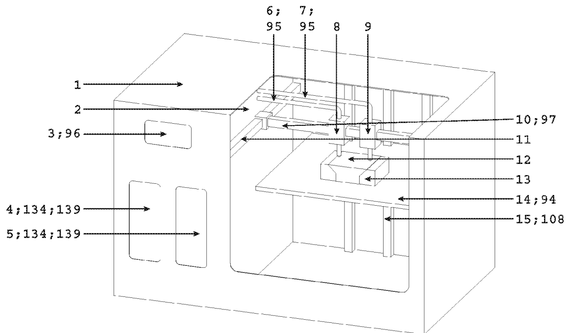
Fig. 1: Extrusionsbasierter 3D-Drucker (schematisch)
