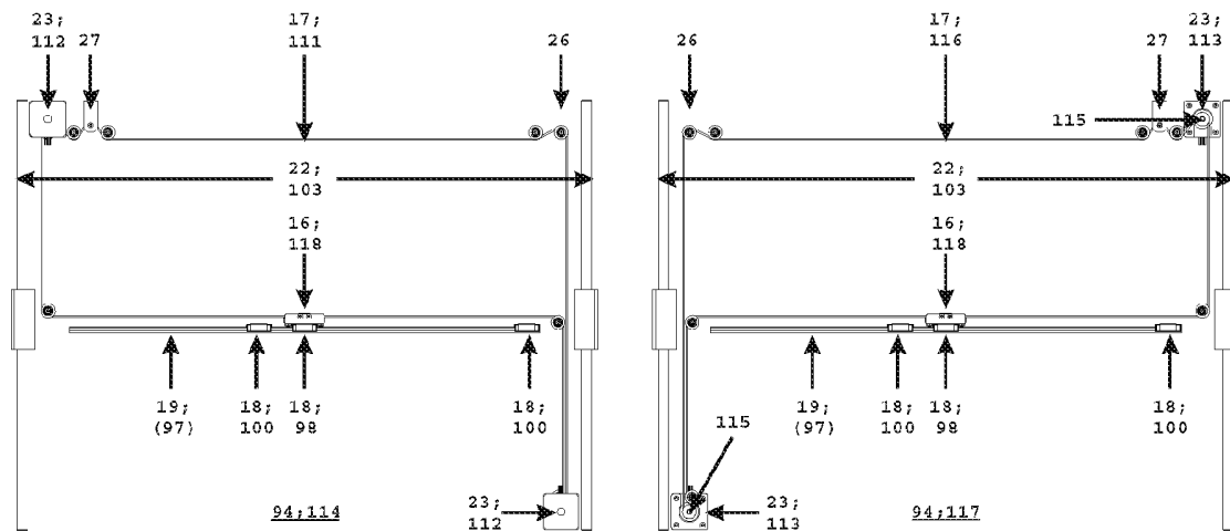
Fig. 4: Zahnriemensystem (vereinfacht)
