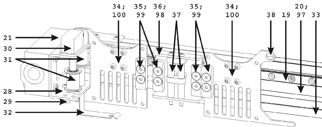
Fig. 5: Andocksystem (Druckköpfe und Zahnriemen nicht dargestellt)
