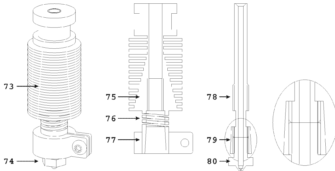
Fig. 14: Schmelzeinheit mit Heizeinheit und Düseneinheit
