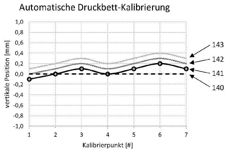
Fig. 11: Automatische Druckbett-Kalibrierung
