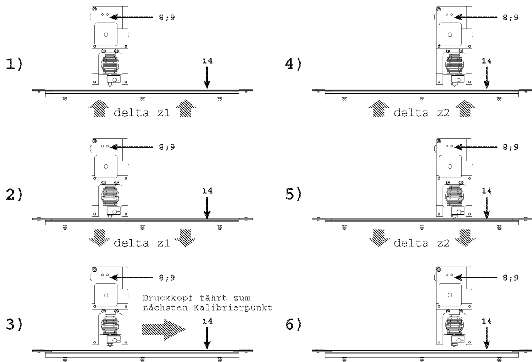
Fig. 10: Automatische Druckbett-Kalibrierung
