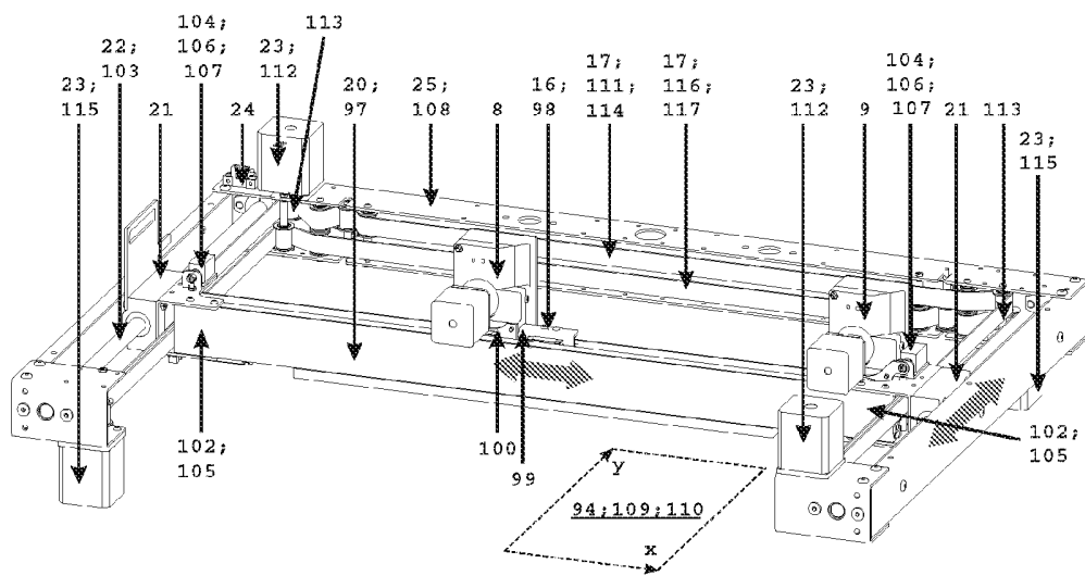
Fig. 2: Horizontales Positioniersystem (Blick von vorn)
