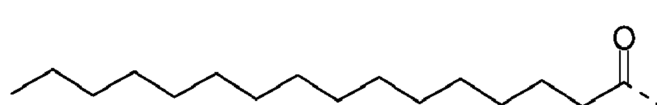
Palmitoyl (Pam)
