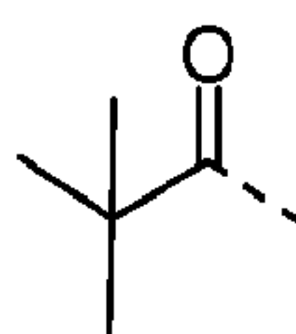
Trimethylacetyl
