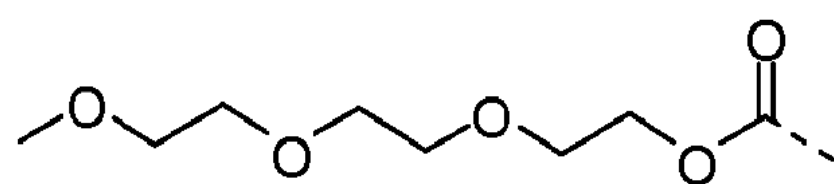
mdPEG3
