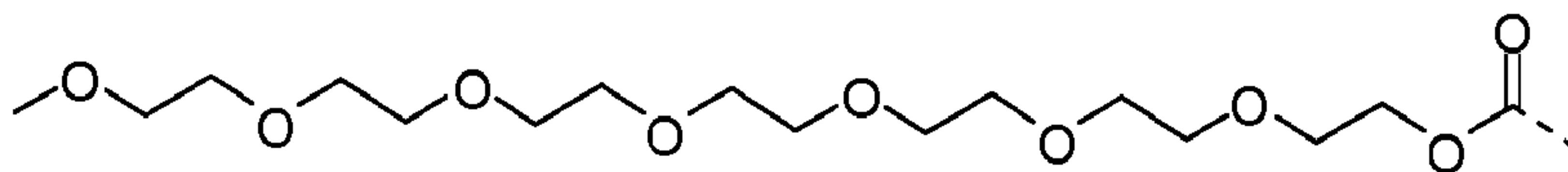
mdPEG7
