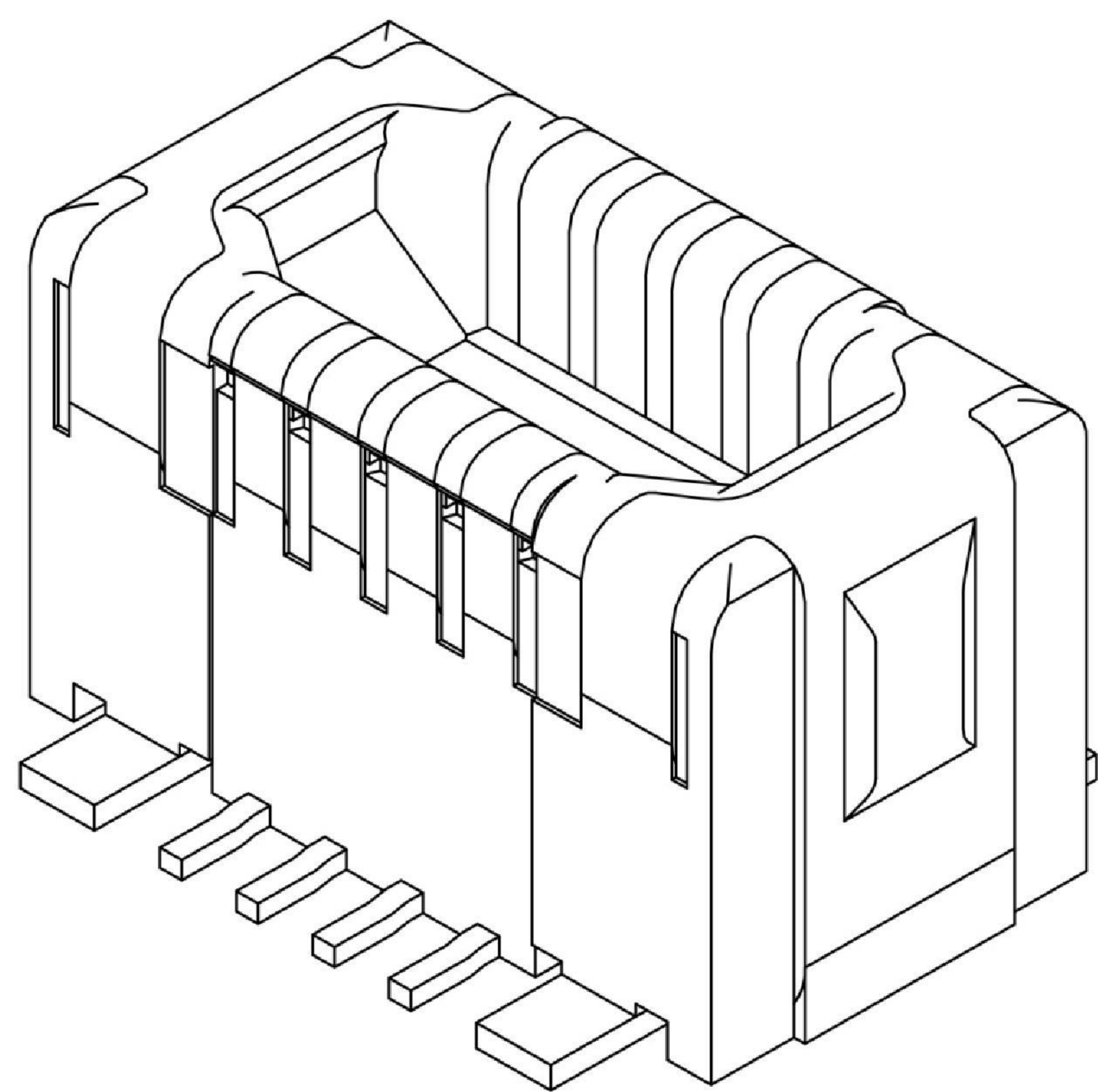
【立體圖 4】
