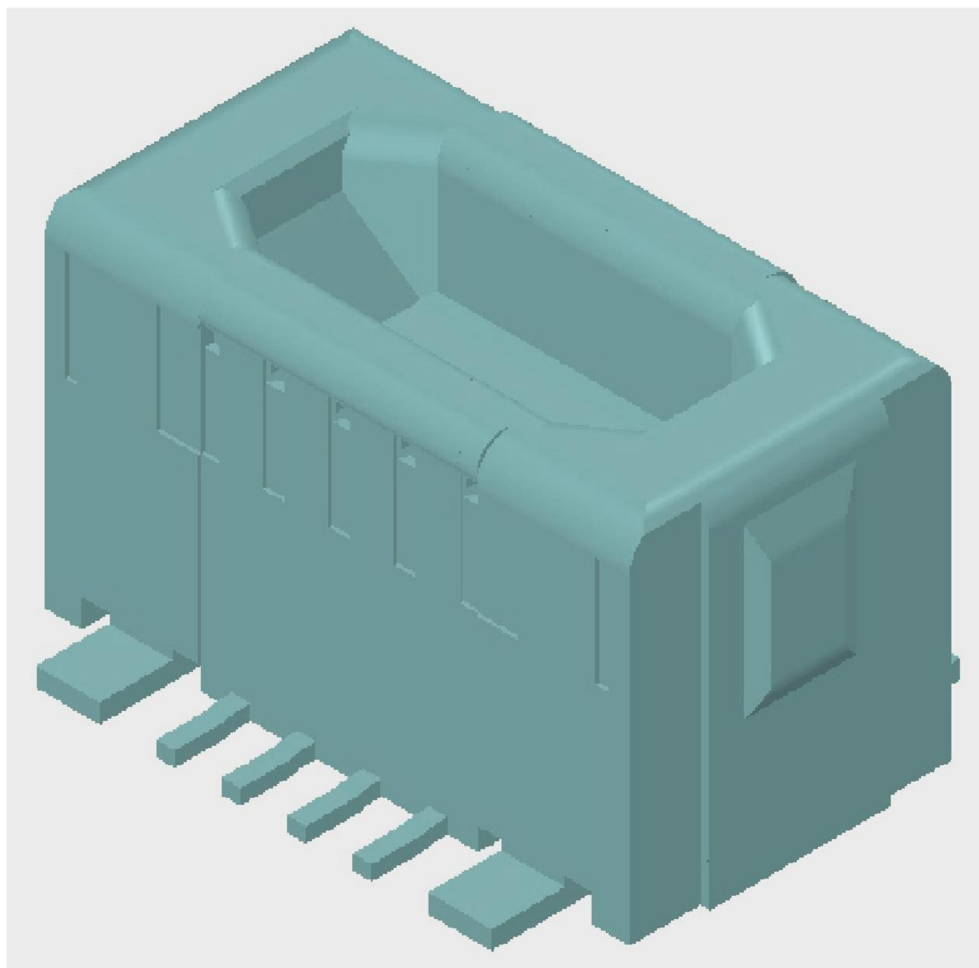
【參考立體圖 1】
