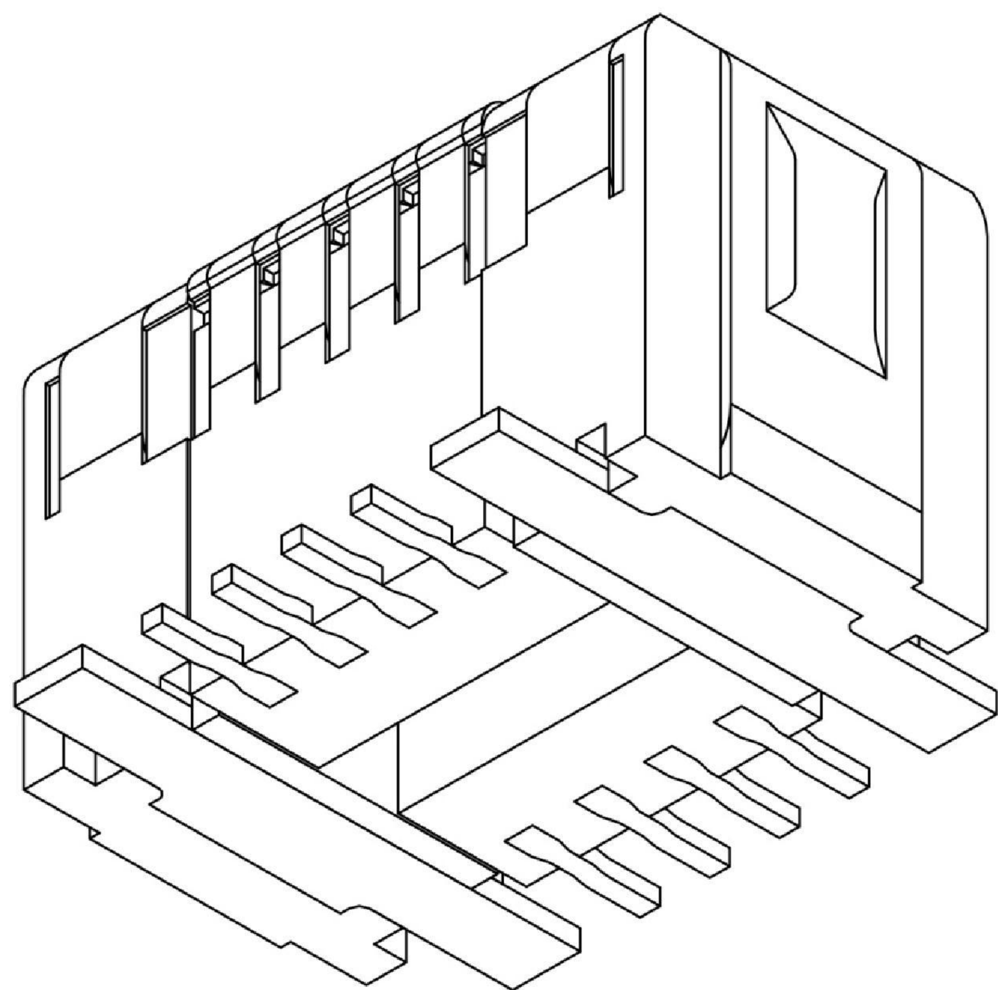
【立體圖 2】
