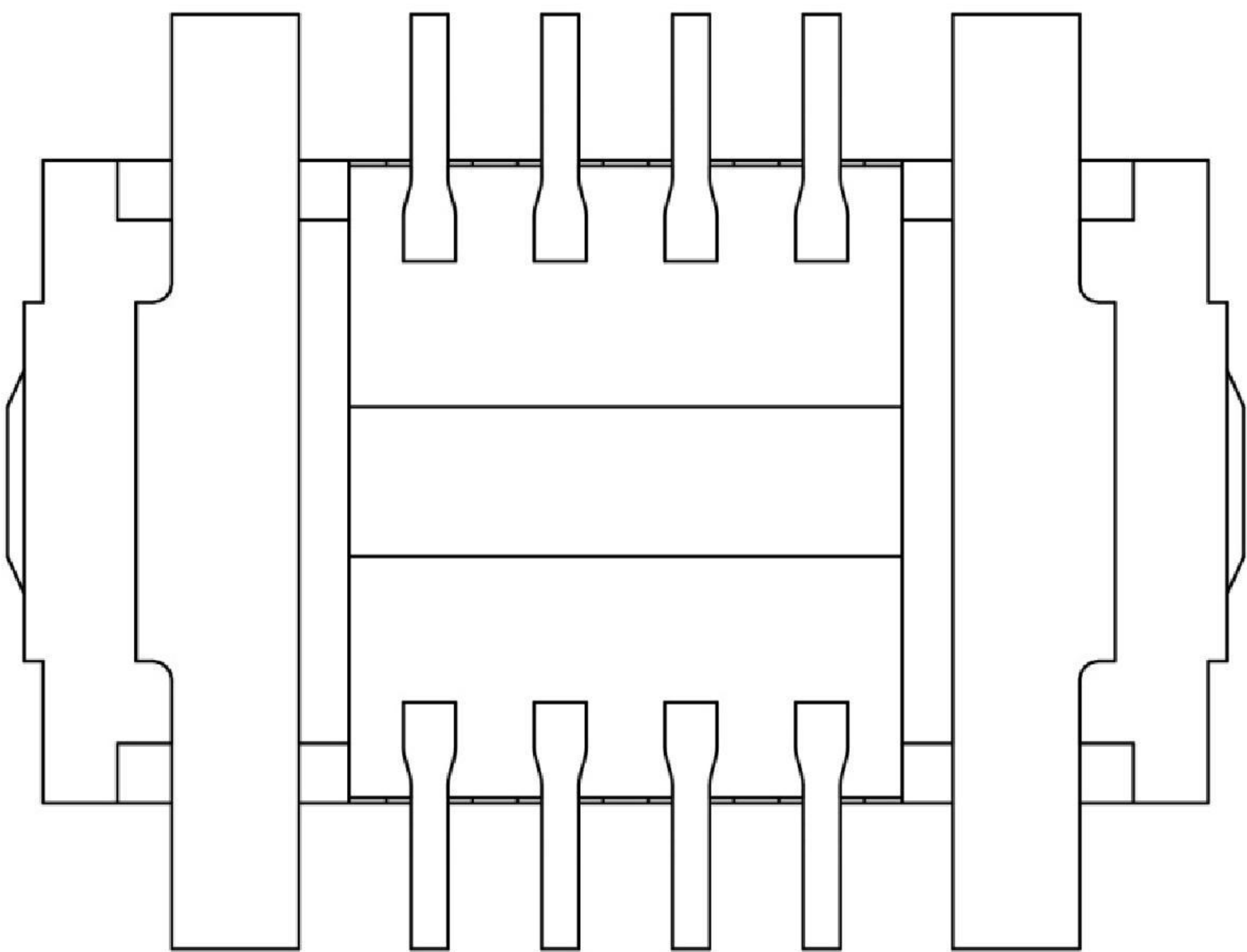
【仰視圖】
