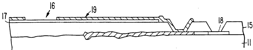
FIG. 3D(1)
