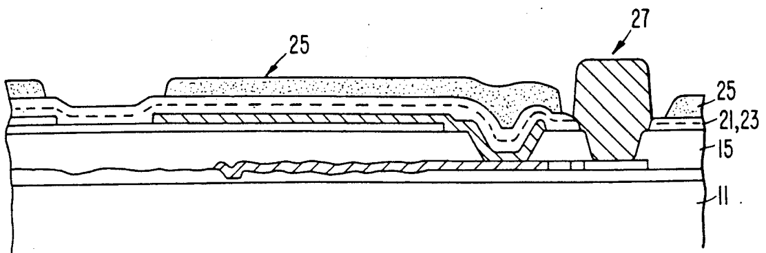
FIG. 3E(2)
