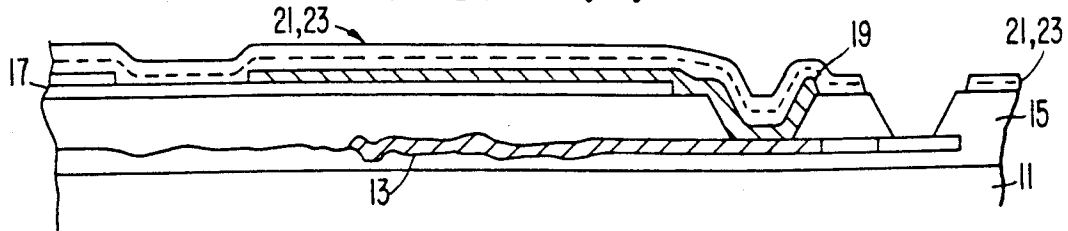
FIG. 3D(2)
