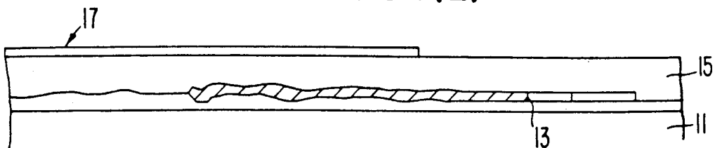
FIG. 3B(2)
