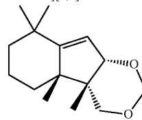
(4aS, 4bR, 9aS)-4a, 4b, 8, 8-tetramethyl-4, 4a, 4b, 5, 6, 7, 8, 9a-octahydroindeno[2, 1-d][1, 3]dioxine
