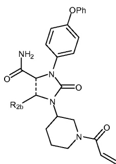
(XVIa)
