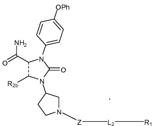
(IVa)
