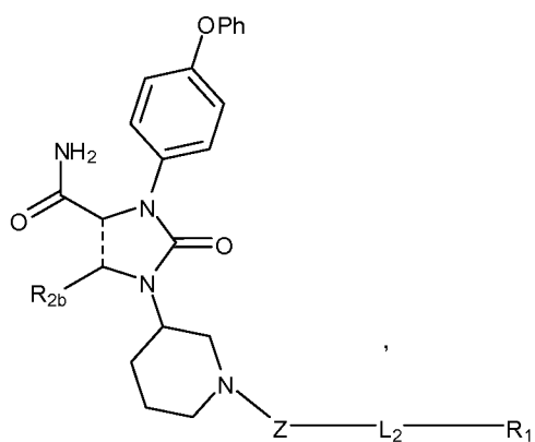
(Va)
