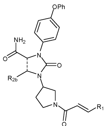
(IXa)
