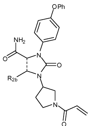
(XVa)
