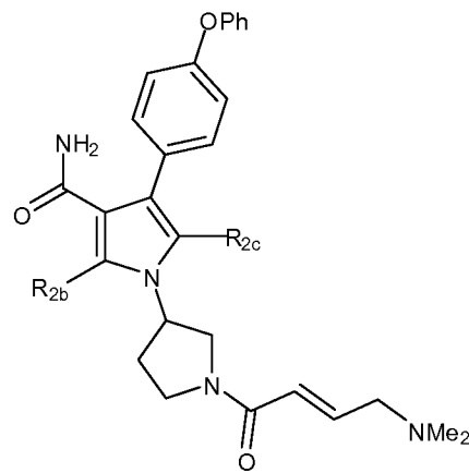
(XVIIIb)
