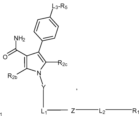
(IIb)
