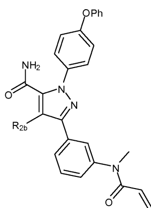
(XVIIc)
