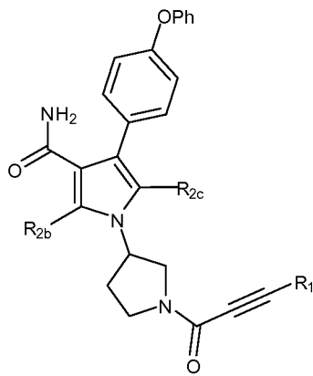
(XIIb)
