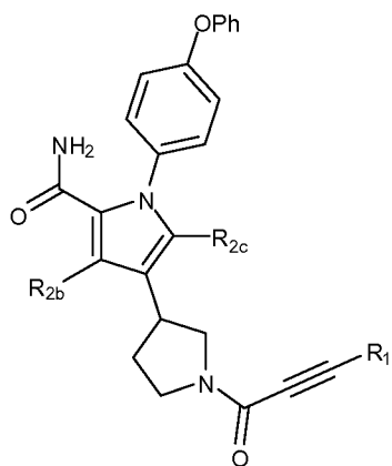
(XIId)
