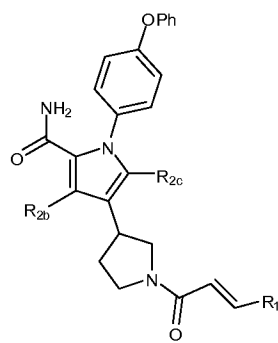
(IXd)
