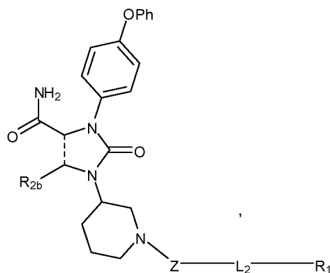
(Va)
