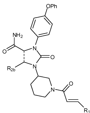
(Xa)
