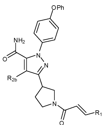
(IXc)
