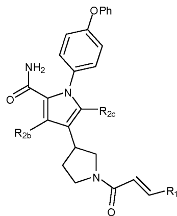
(IXd)
