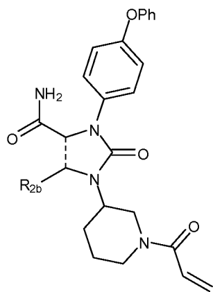
(XVIa)
