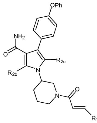
(Xb)
