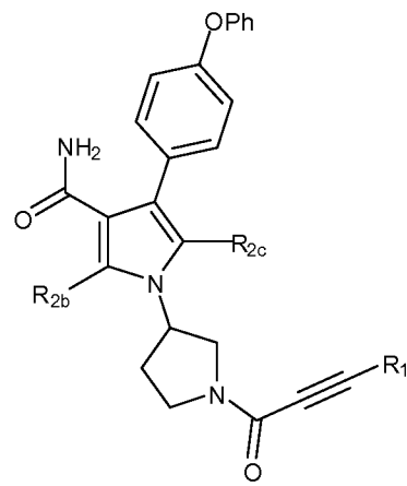
(XIIb)
