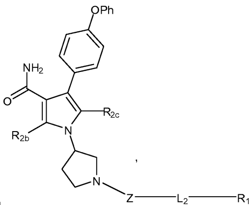
(IVb)
