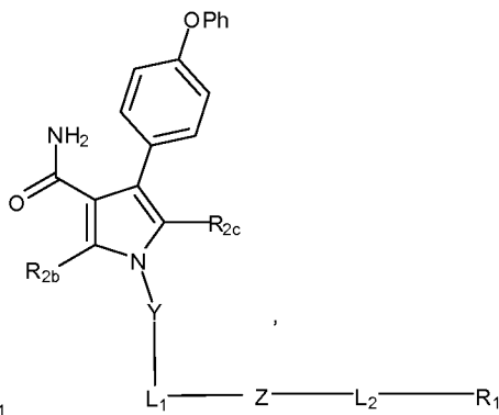
(IIIb)
