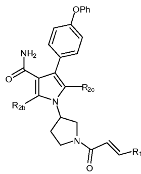
(IXb)
