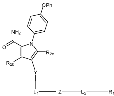
(IIId)
