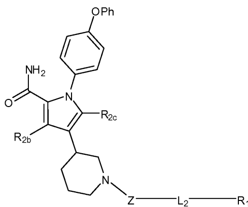
(Vb)
