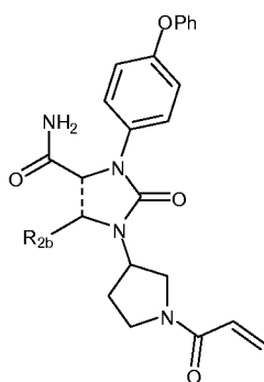
(XVa)
