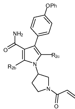
(XVb)
