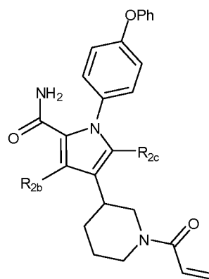
(XVIId)
