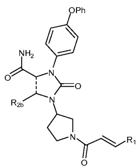
(IXa)
