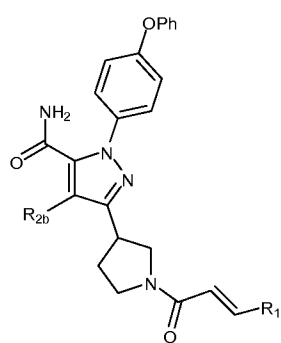
(IXc)
