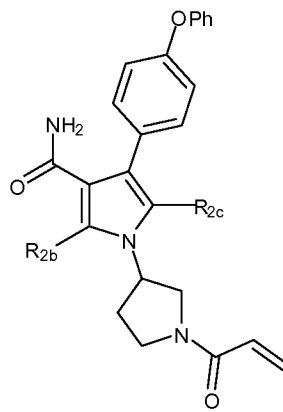
(XVb)
