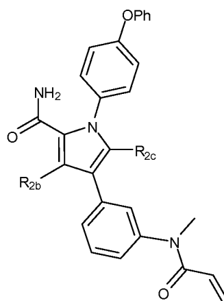
(XVIIId)
