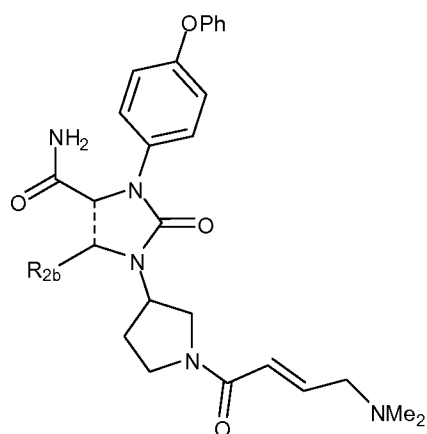
(XVIIIa)
