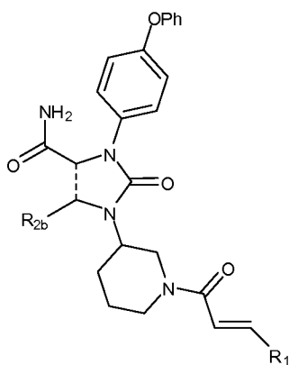
(Xa)
