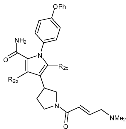
(XVIIId)
