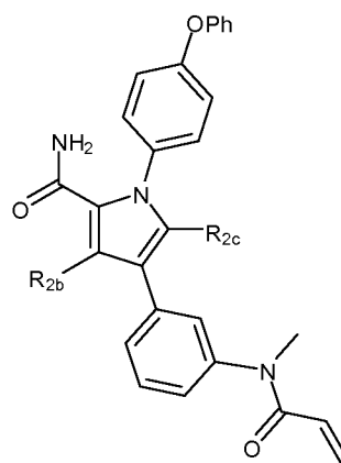
(XVIIId)
