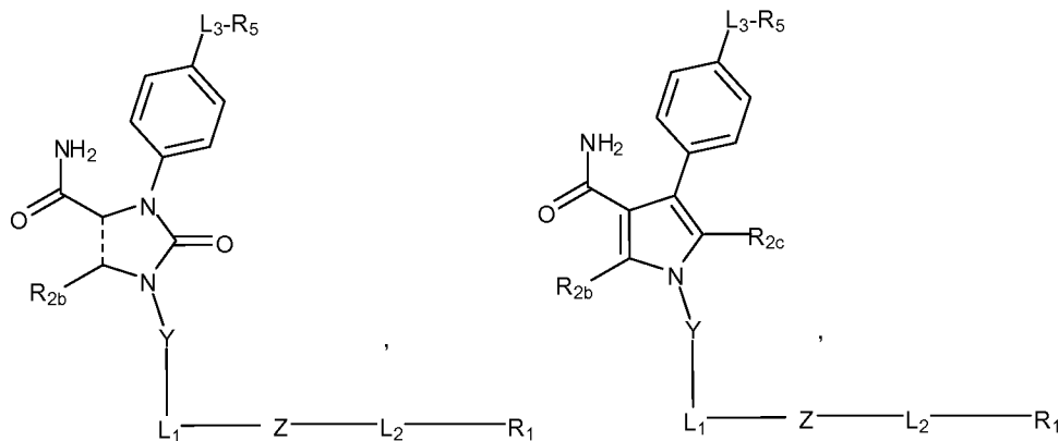
(IIb)
