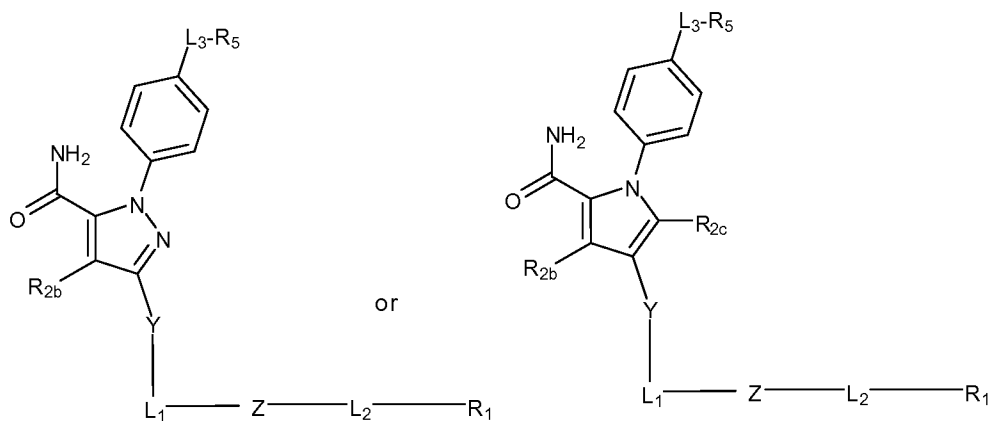
(IIa)
