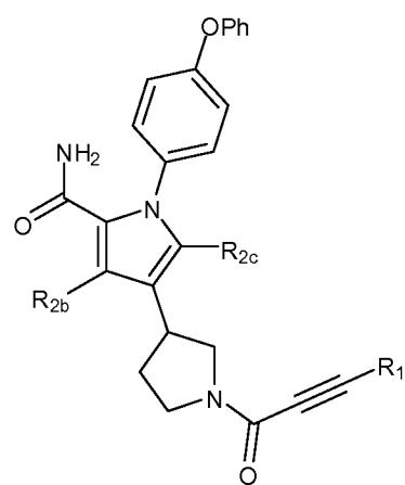
(XIId)
