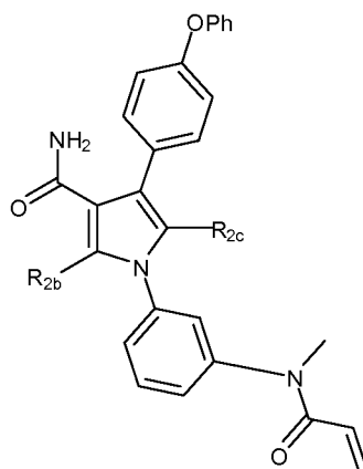
(XVIIb)
