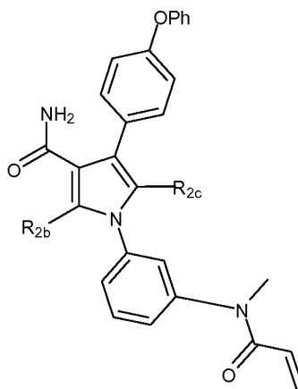
(XVIIb)
