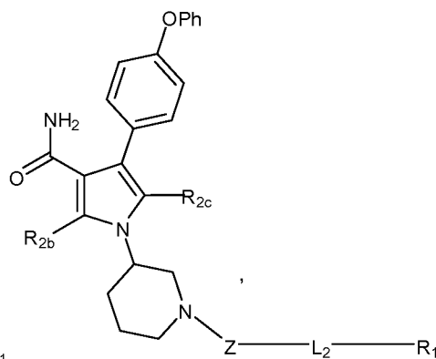
(Vb)
