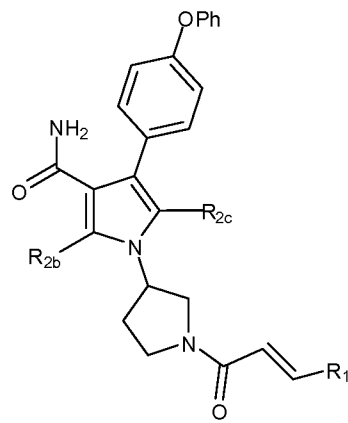
(IXb)
