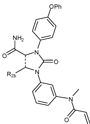
(XVIIa)
