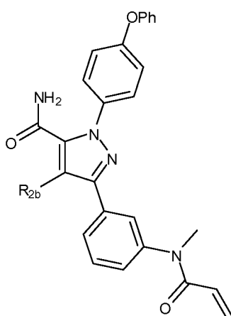
(XVIIc)
