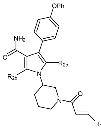
(Xb)
