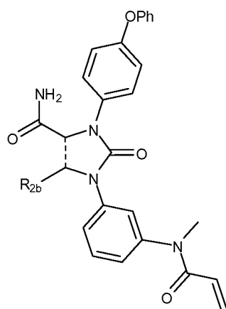
(XVIIa)
