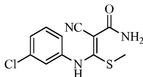
3-((3-chlorophenyl)amino)-2-cyano-3-(methylthio)acrylamide
