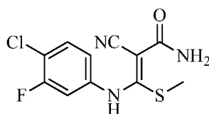
3-((4-chloro-3-fluorophenyl)amino)-2-cyano-3-(methylthio)acrylamide
