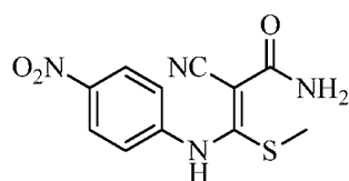
2-cyano-3-(methylthio)-3-((4-nitrophenyl)amino)acrylamide
