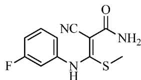
2-cyano-3-((3-fluorophenyl)amino)-3-(methylthio)acrylamide
