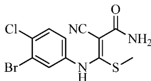
3-((3-bromo-4-chlorophenyl)amino)-2-cyano-3-(methylthio)acrylamide
