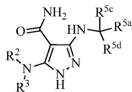
(XVI-a)
