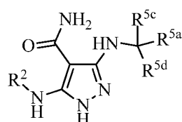
(XIV-c)
