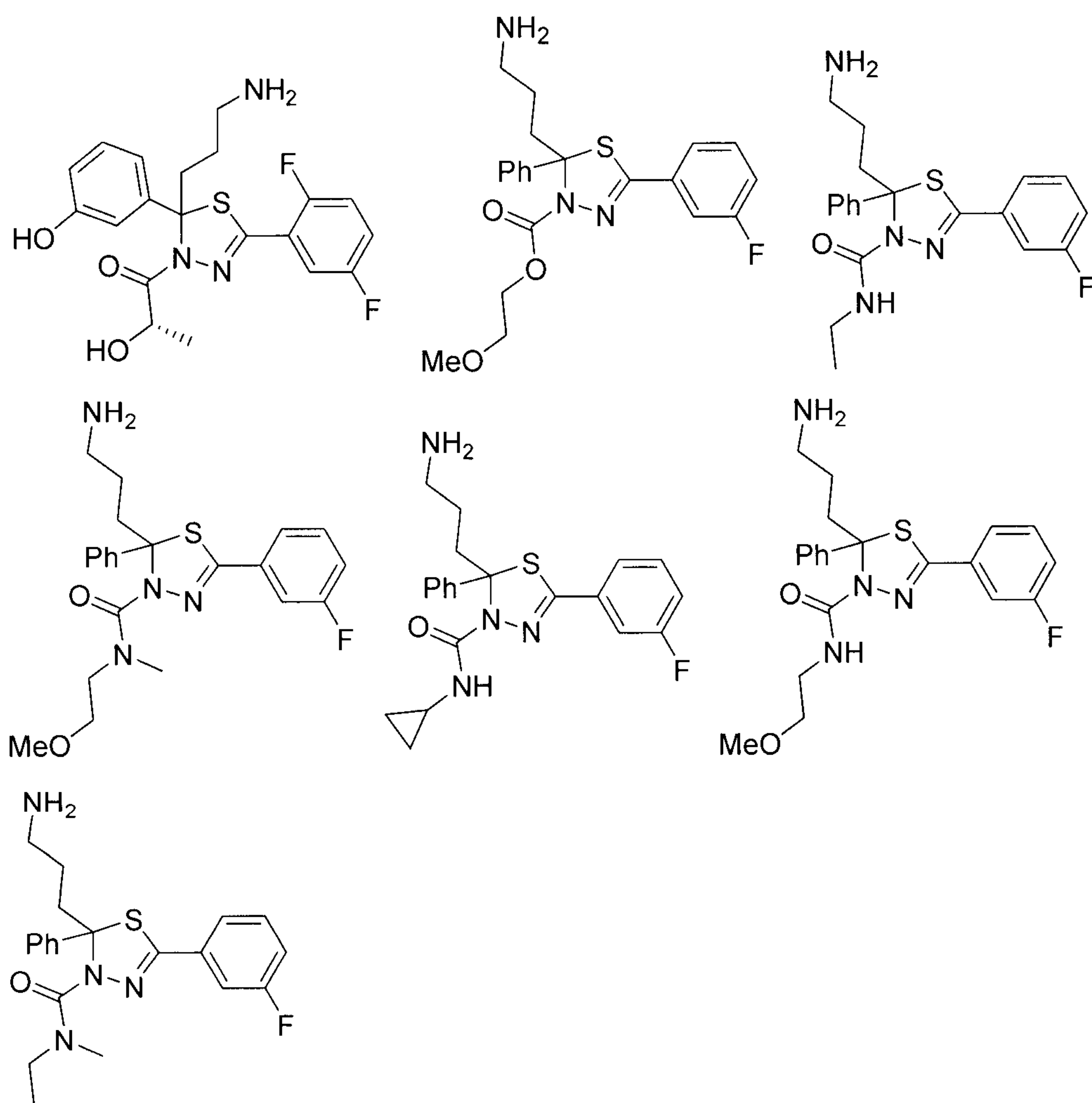
(Diastereomer A)
