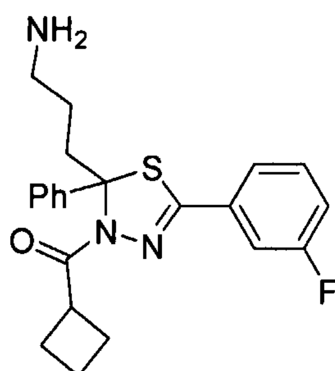
(2-(3-Aminopropyl)-5-(3-fluorophenyl)-2-phenyl-1,3,4-thiadiazol-3(2H)-yl)(cyclobutyl)methanone
