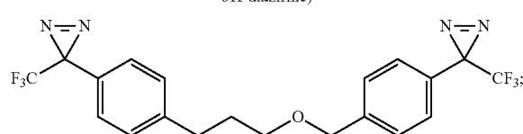
3-(trifluoromethyl)-3-(4-(2-((4-(3-(trifluoromethyl)-3H-diazirin-3-yl)benzyl)oxy)propyl)phenyl)-3H-diazirine
