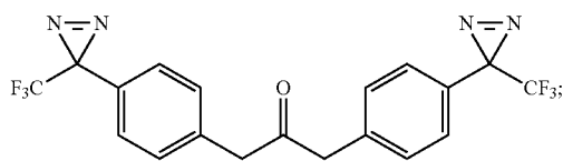
1,3-bis(4-(3-(trifluoromethyl)-3H-diazirin-3-yl)phenyl)propan-2-one
