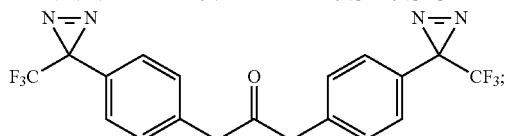
1,3-bis(4-(3-(trifluoromethyl)-3H-diazirin-3-yl)phenyl)propan-2-one
