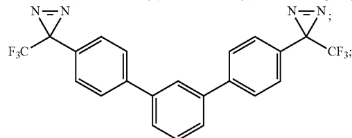
4,4''-bis(3-(trifluoromethyl)-3H-diazirin-3-yl)-1,1':3',1''-terphenyl
