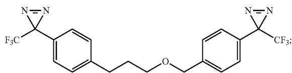
3-(trifluoromethyl)-3-((4-(3-(trifluoromethyl)-3H-diazirin-3-yl)benzyl)oxy)propyl)phenyl-3H-diazirine
