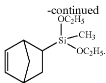
bicyclo[2.2.1]hept-5-en-2-yl(triethoxy)silane (TESNB)
