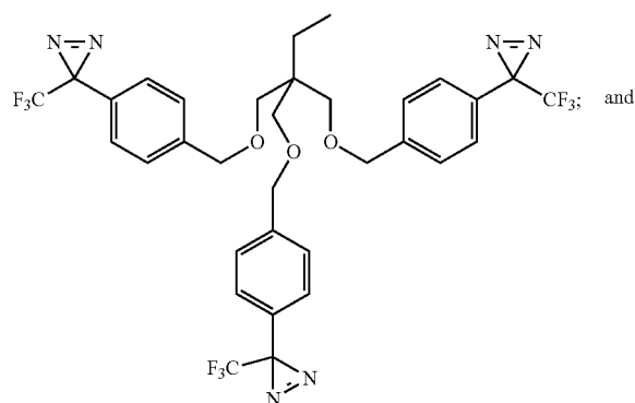
3,3'-(((2-ethyl-2-(((4-(3-(trifluoromethyl)-3H-diazirin-3-yl)benzyl)oxy)methyl)propane-1,3-diyl)bis(oxy))bis(methylene))bis(4,1-phenylene))bis(3-(trifluoromethyl)-3H-diazirine)
