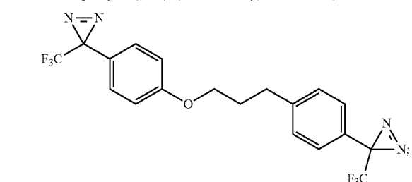
3-(trifluoromethyl)-3-(4-(3-(4-(3-(trifluoromethyl)-3H-diazirin-3-yl)phenoxy)propyl)phenyl)-3H-diazirine
