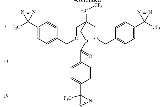
3,3'-(((2-(2-(perfluoroethyl)-2-(((4-(3-(trifluoromethyl)-3H-diazirin-3-yl)benzyl)oxy)methyl)propane-1,3-diyl)bis(oxy))bis(methylene))bis(4,1-phenylene))bis(3-(trifluoromethyl)-3H-diazirine)
