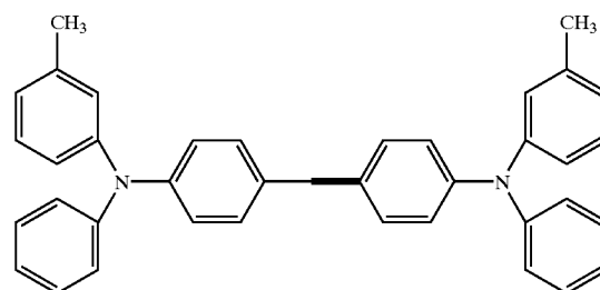
TPD
