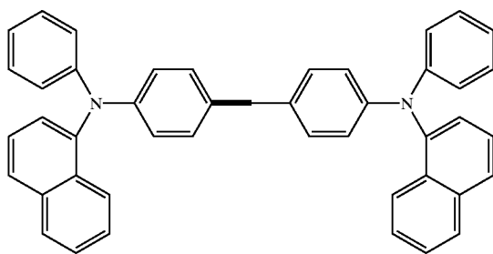
\alpha -NPD
