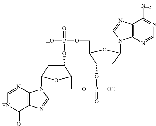
c-(dAMP-dIMP)
