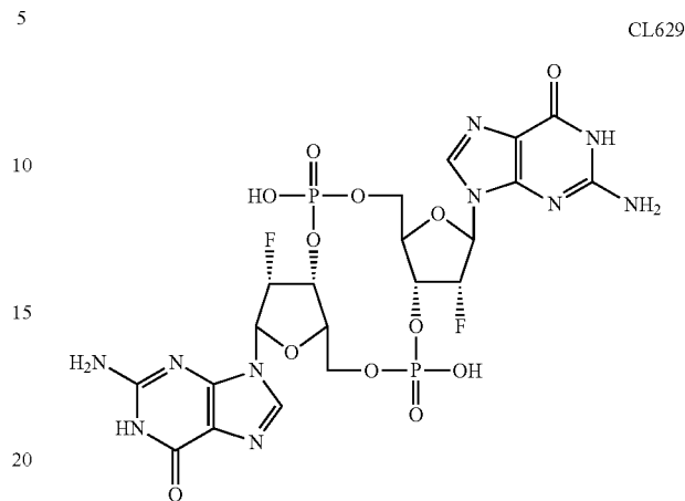
c-di(2'FdGMP)
