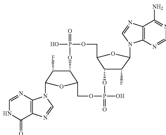
c-(2'FdAMP-2'FdIMP)
