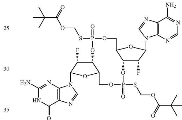
c-[2'FdGMP(S)-2'FdAMP(S)](POM) 2
