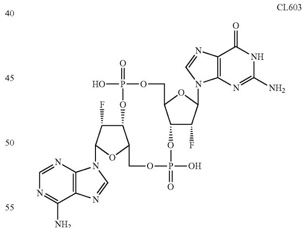
c-(2'FdGMP-2'FdAMP)
