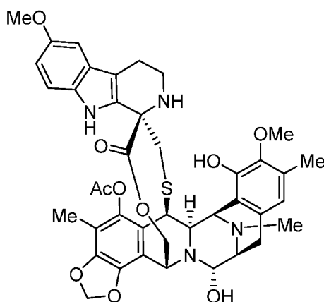
lurbinectedin
