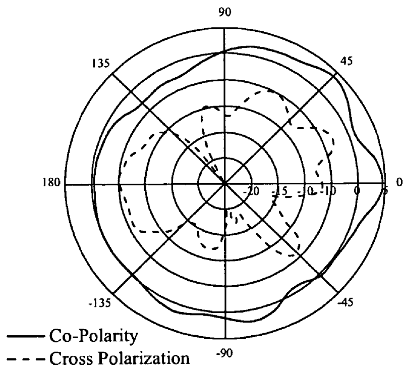
H-Plane
