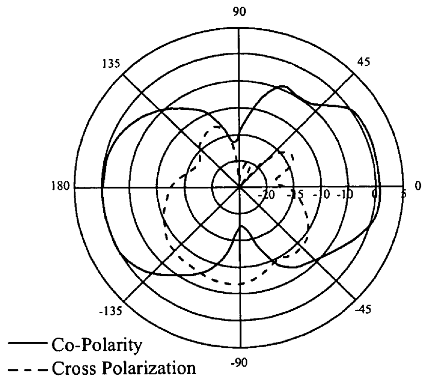
E-Plane
