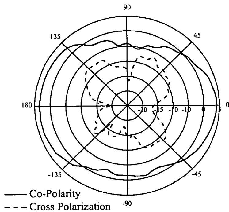
H-Plane
