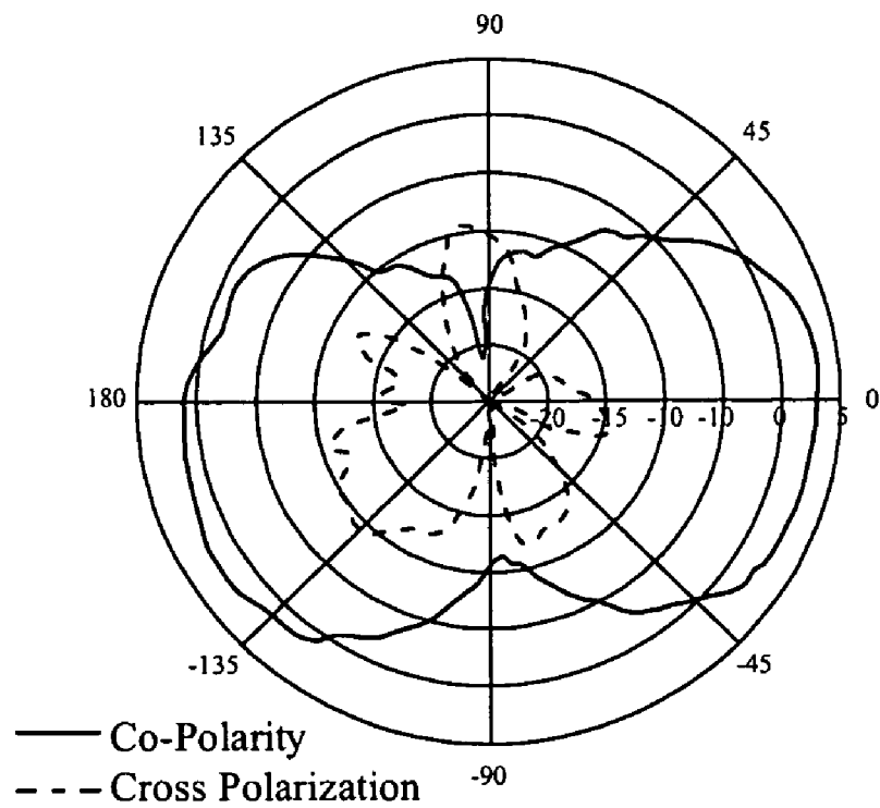
E-Plane
