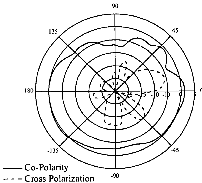
H-Plane
