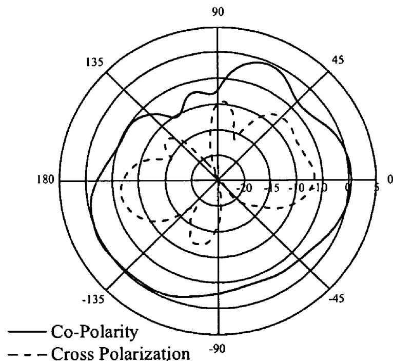
H-Plane
