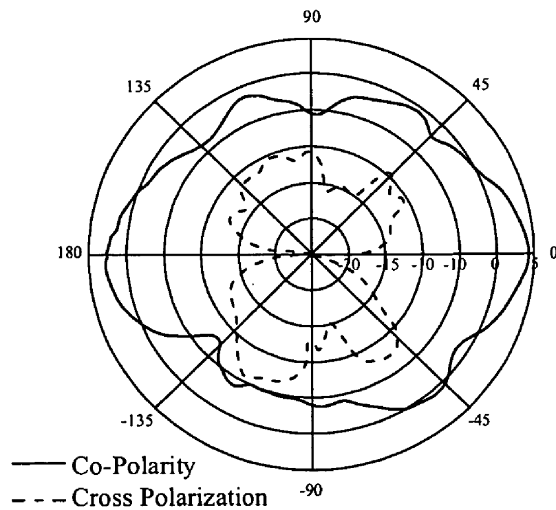
H-Plane
