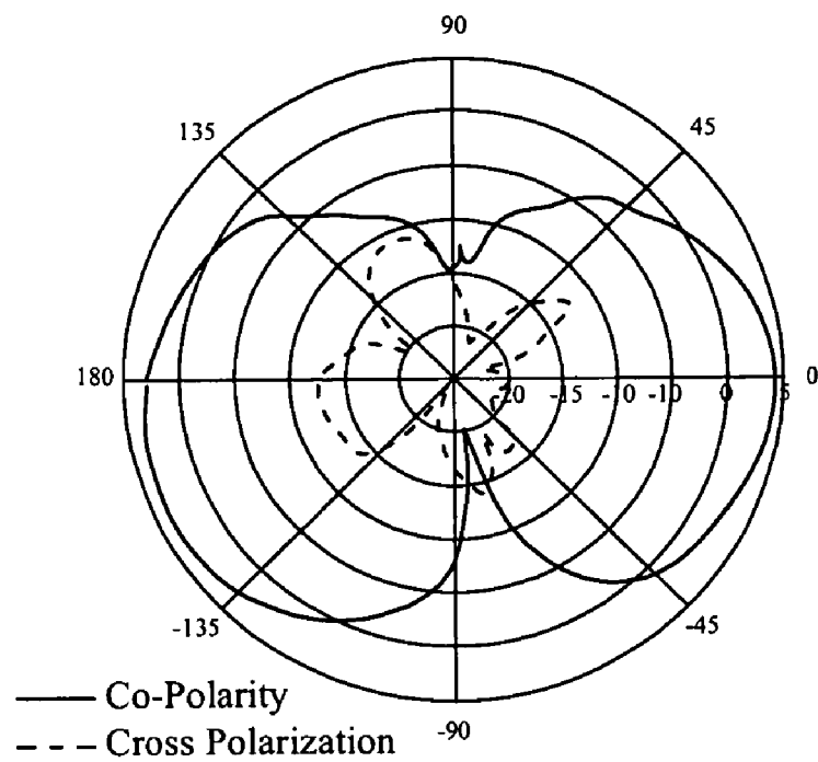
E-Plane
