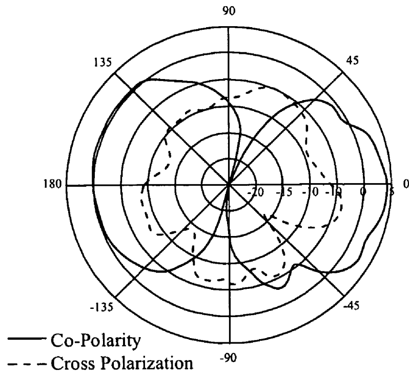
E-Plane
