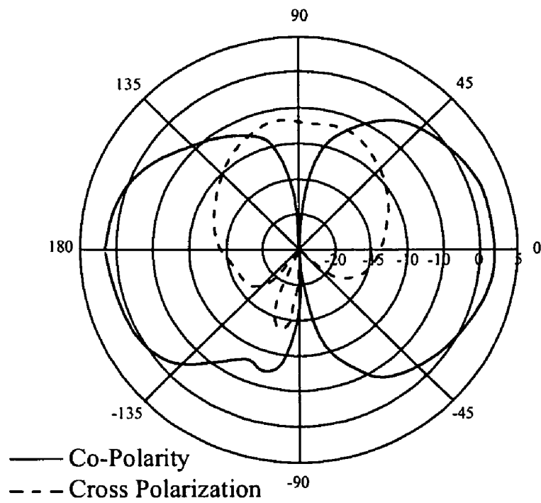
E-Plane
