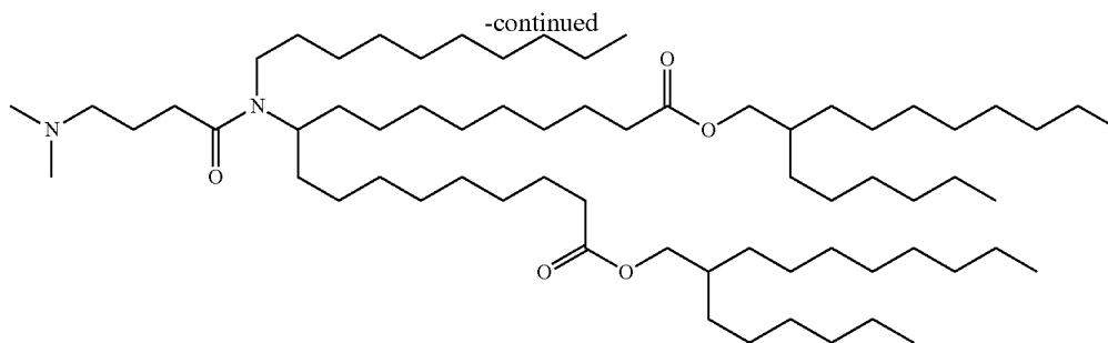
I-38
