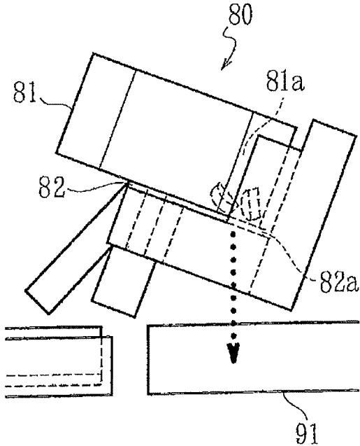
FIG. 13(b)
