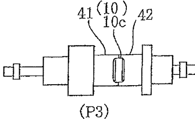
FIG.4 (g)
