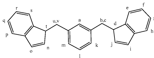
1,3-bis((1 H -inden-1-yl)methyl)benzene
