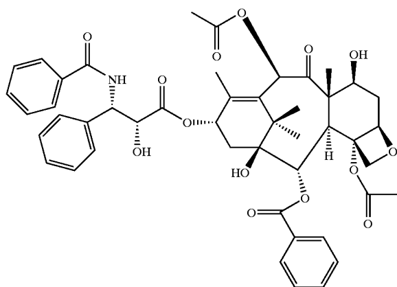
Taxol (paclitaxel)
