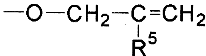
Formule (F)
