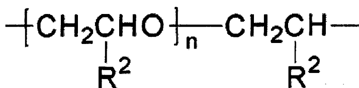
Formule (B)
