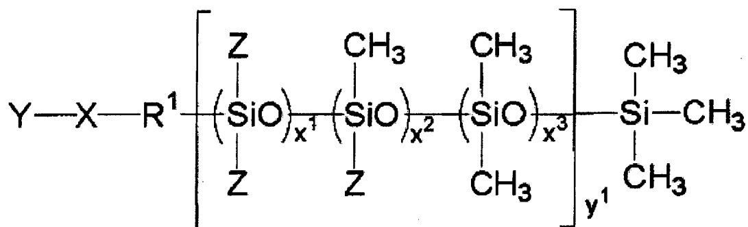
Formule (A)
