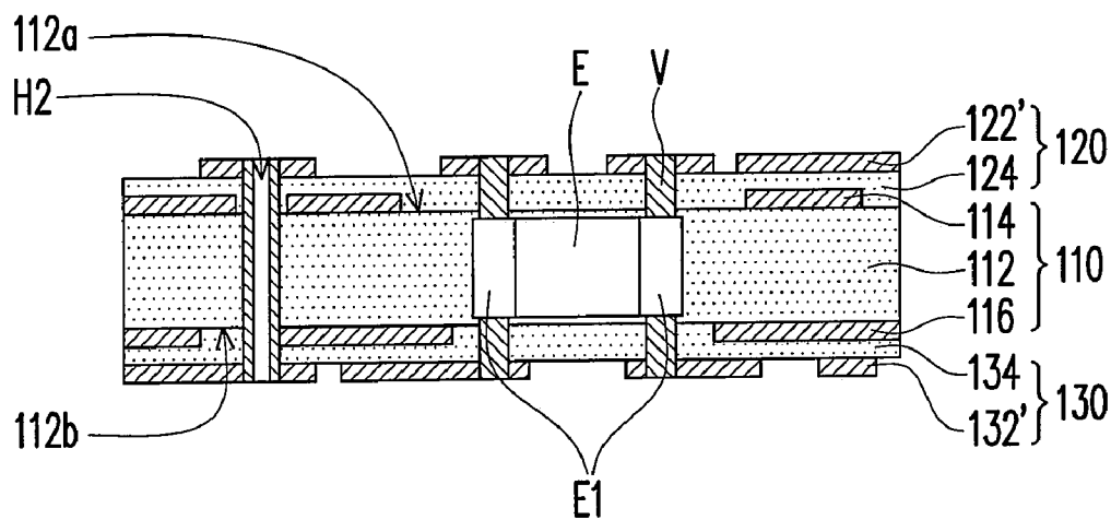
FIG. 1E(PRIOR ART)
