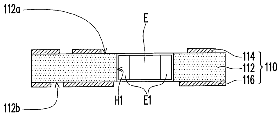
FIG. 1B(PRIOR ART)
