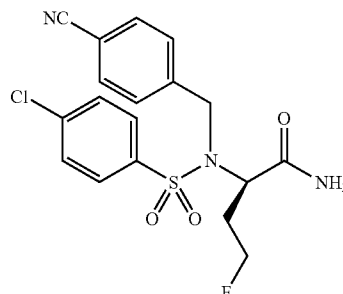
(2R)-2-[(4-Chlorobenzenesulfonyl)-(4-cyanobenzyl)-amino]-4-fluorobutyramide (Example 360)
