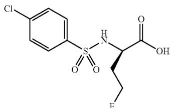
(2R)-2-(4-Chlorobenzenesulfonylamino)-4-fluorobutanoic acid
