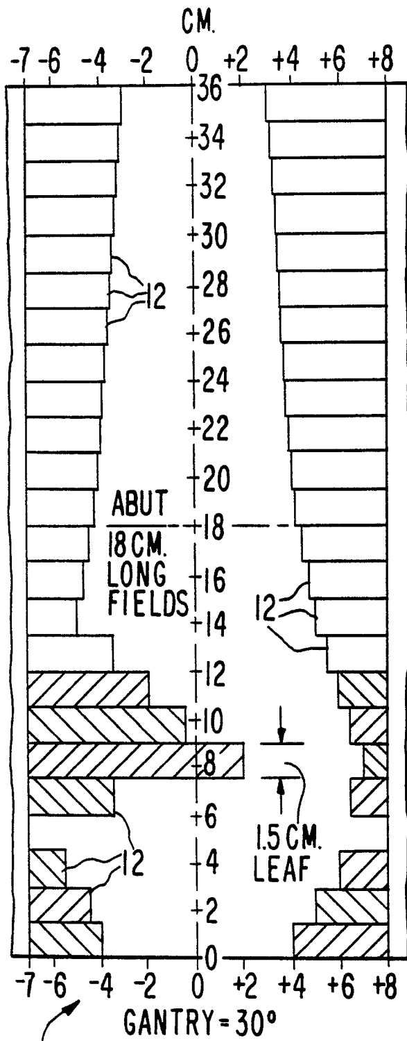
RIGHT OBLIQUE
