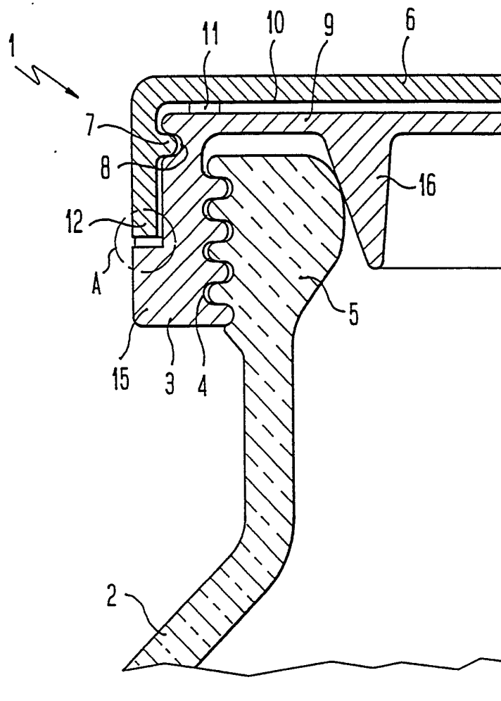
Seitenansicht A
