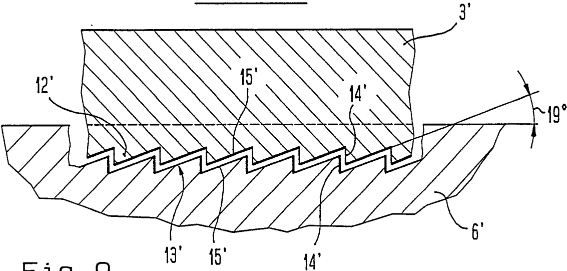
5/6 Schnitt A-A
