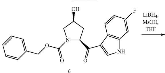
Scheme VI
