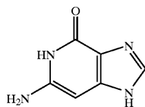
3-deaza-Guanine
