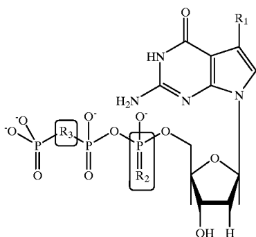
7-Substituted-7-Deaza-dGTP
