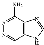
2-aza-3-deaza-Adenine
