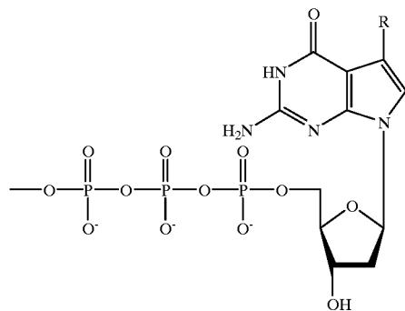
7-deaza-dGTP
