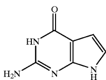
7-deaza-Guanine
