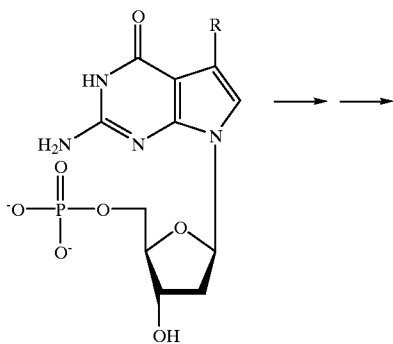
7-deaza-dGMP
