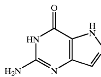
8-Aza-9-deaza-Guanine
