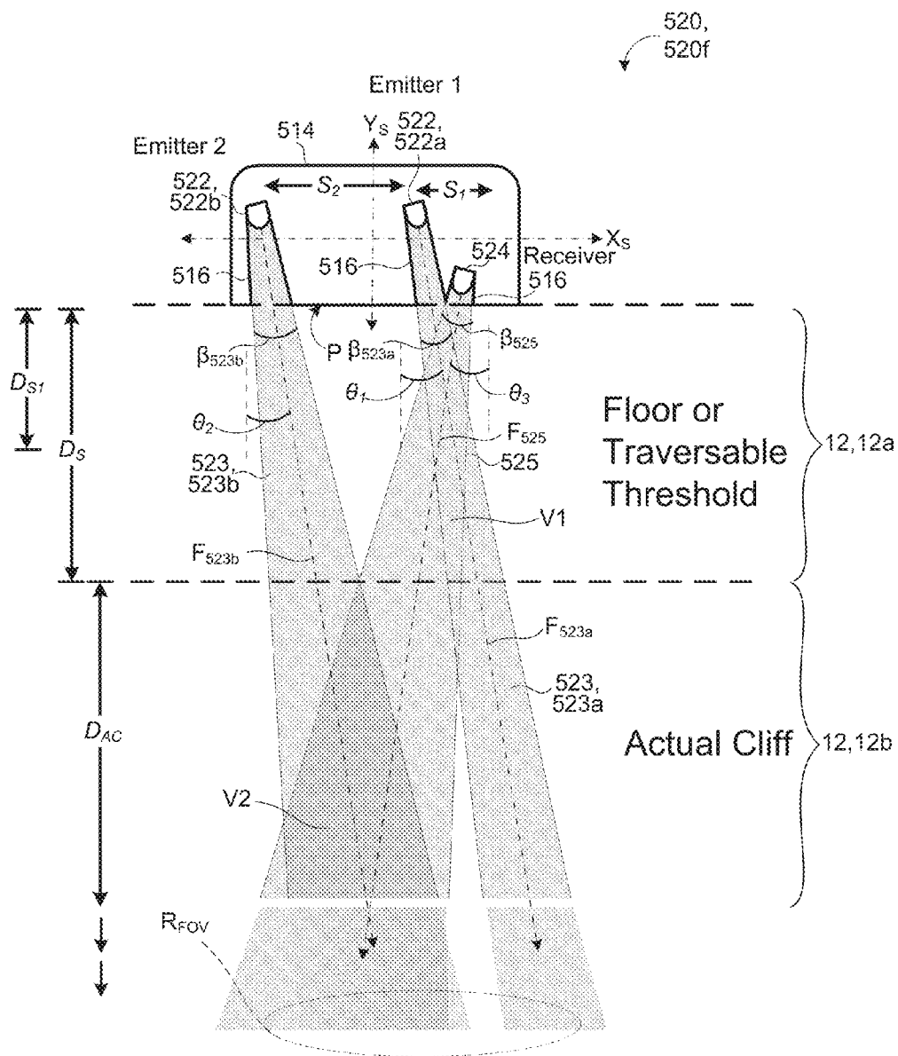
FIG. 9B
