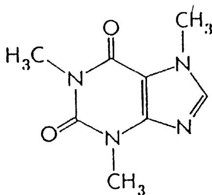
Caffeine
