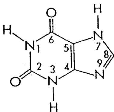
Xanthine
