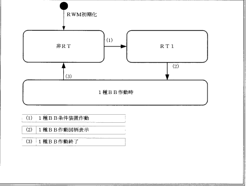
(2) RT 遷移図
