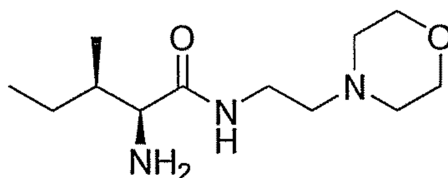
(2S,3R)-2-amino-3-methyl-N-(2-morpholinoethyl)pentanamide
