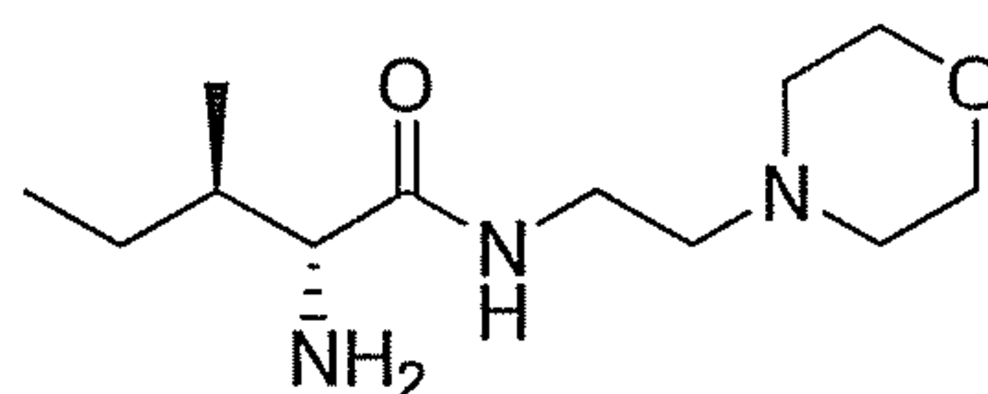
(2R,3R)-2-amino-3-methyl-N-(2-morpholinoethyl)pentanamide
