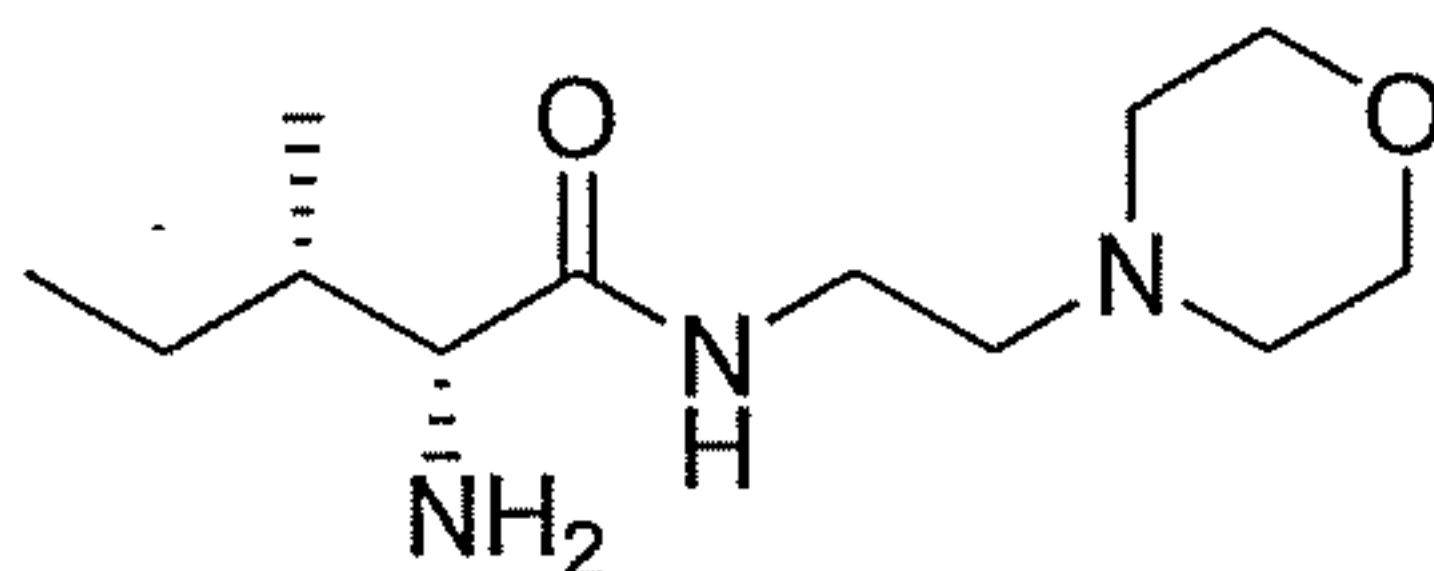
(2 R ,3 S )-2-amino-3-methyl- N -(2-morpholinoethyl)pentanamide
