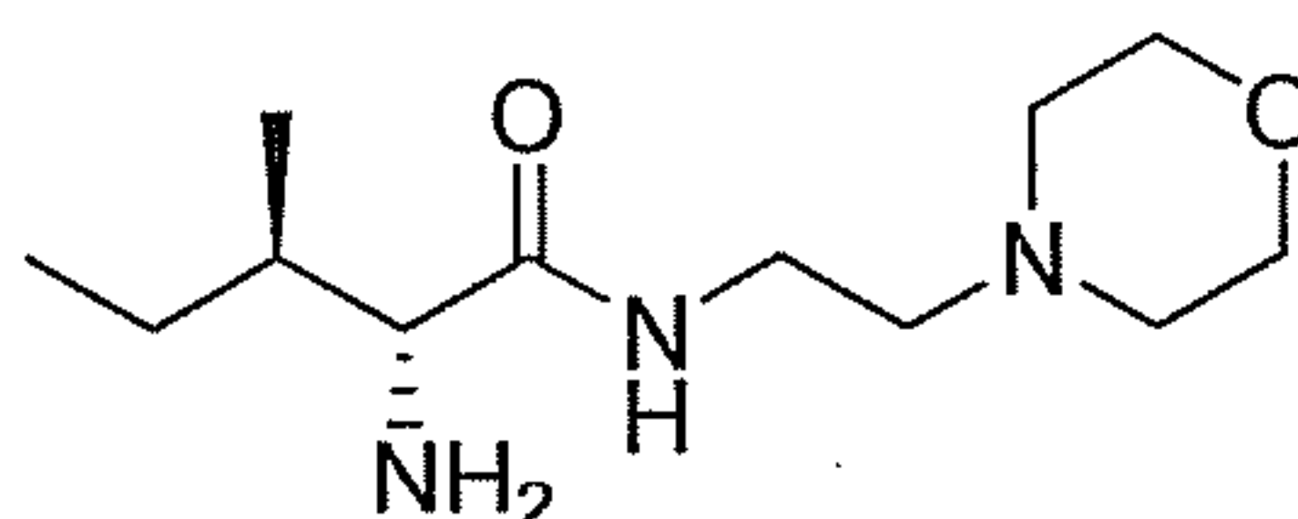
(2R,3R)-2-amino-3-methyl-N-(2-morpholinoethyl)pentanamide
