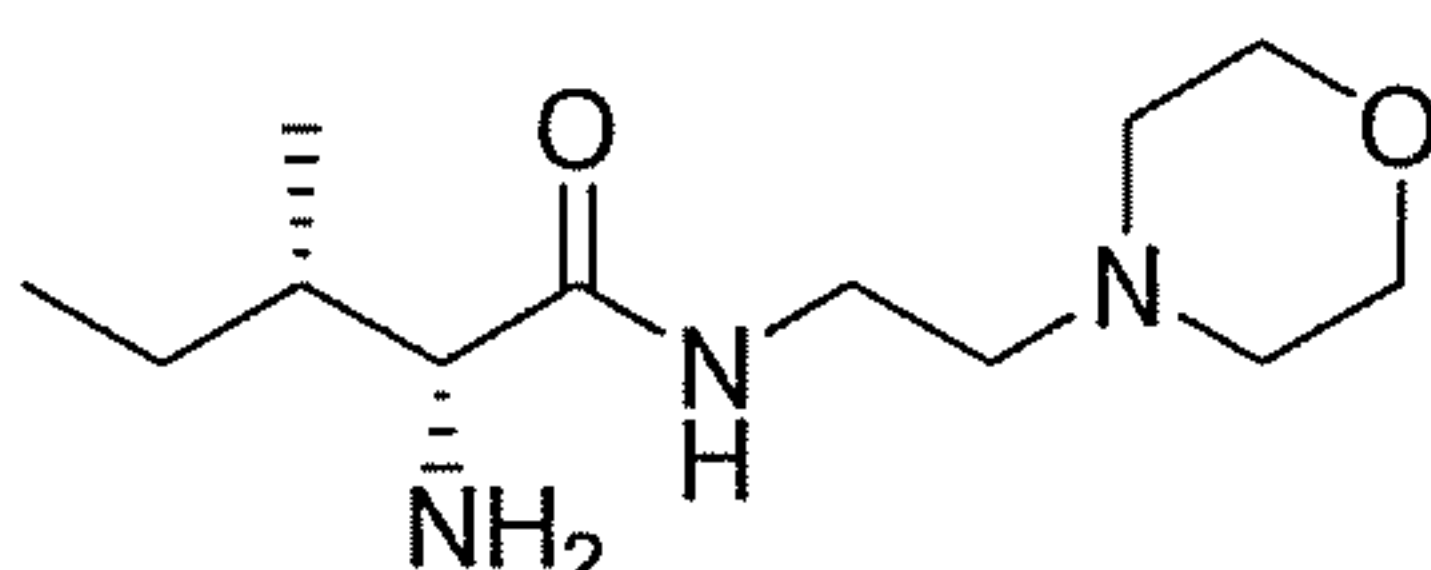
(2R,3S)-2-amino-3-methyl-N-(2-morpholinoethyl)pentanamide
