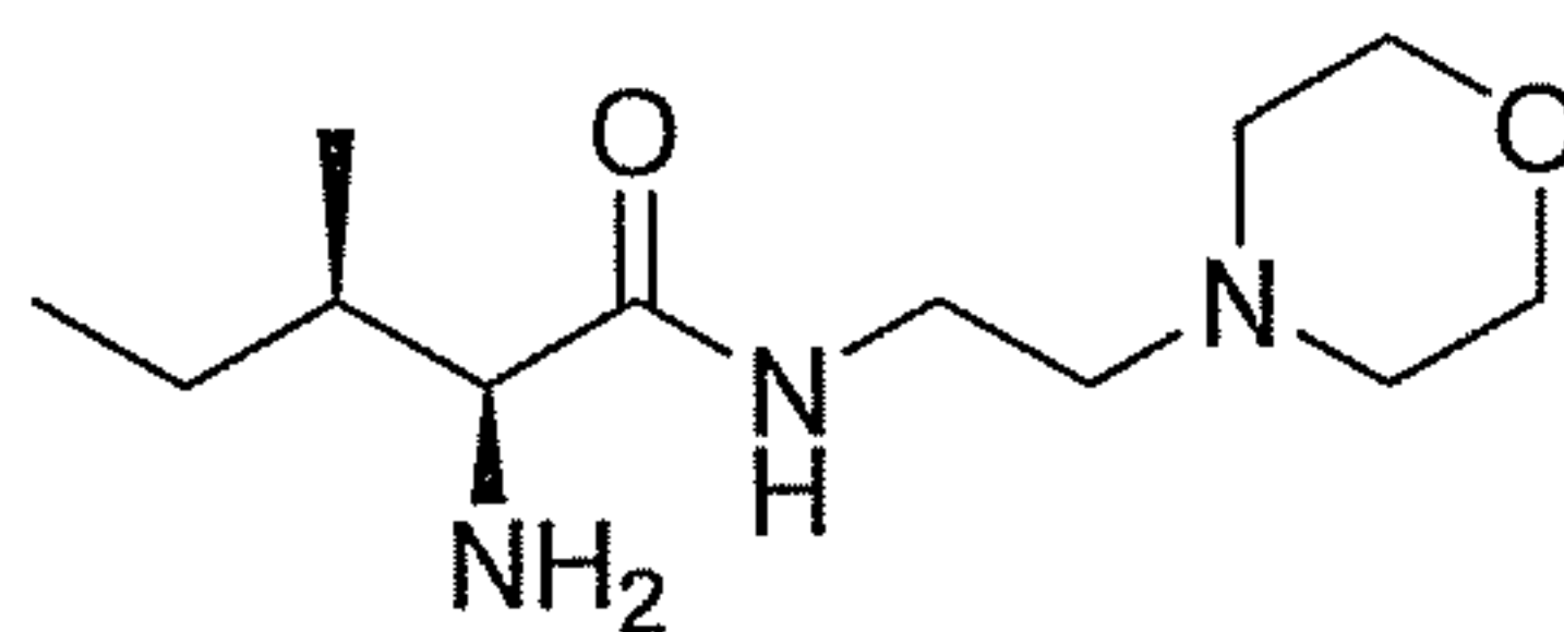
(2 S ,3 R )-2-amino-3-methyl- N -(2-morpholinoethyl)pentanamide
