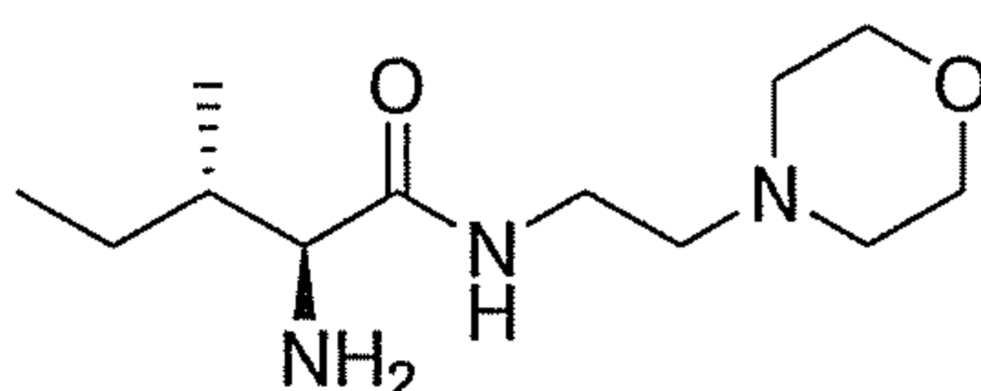
(2S,3S)-2-amino-3-methyl-N-(2-morpholinoethyl)pentanamide
