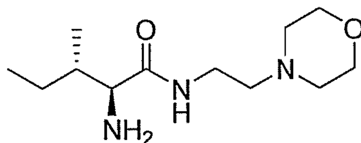
(2S,3S)-2-amino-3-methyl-N-(2-morpholinoethyl)pentanamide
