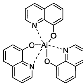
Alq
