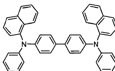
\alpha -NPD
