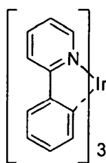
Ir(ppy) 3
