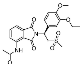
화합물 A
