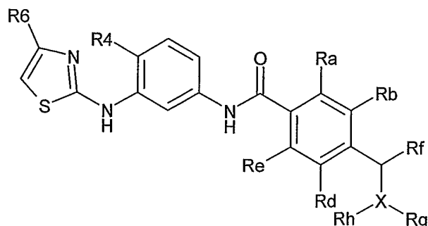
FORMULA II-4
