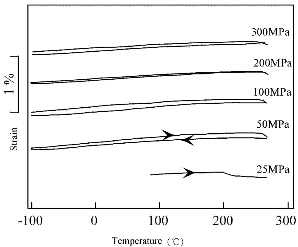
Fig. 4 Ti-22mol%Nb
