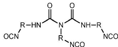
biuret trimer
