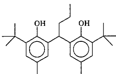
(還元剤 - 2)
