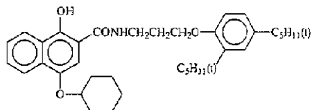
(A-11)
