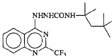
(現像促進剤-1)
