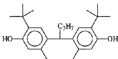
(R-33)
