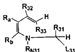
一般式 (3)
