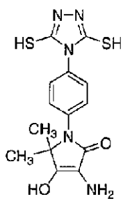
(40)
