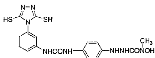
(34)
