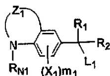
一般式 (1)
