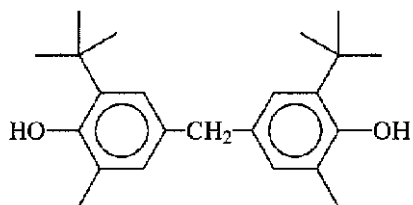
(R-31)
