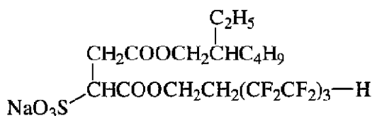
(F-2)
