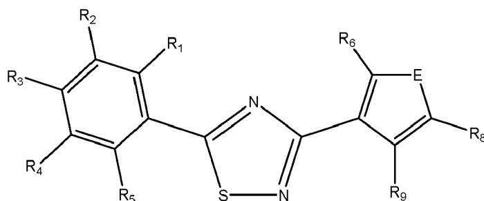
Formula VIIb
