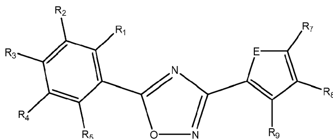
Formula Va
