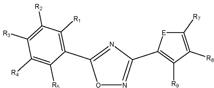
Formula Va
