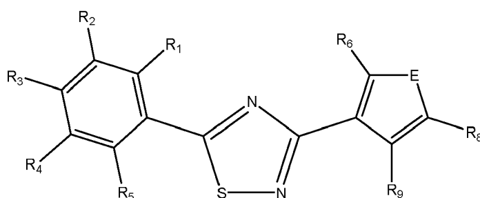
Formula VIIb
