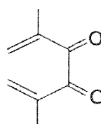
(d) carbonyl group or quinone group
