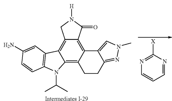
Scheme 18.
