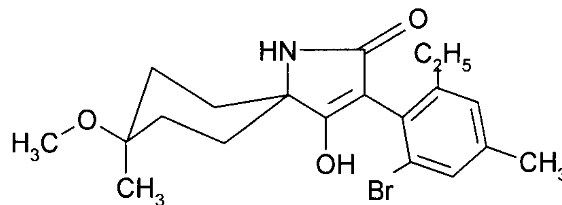
I-a-2
