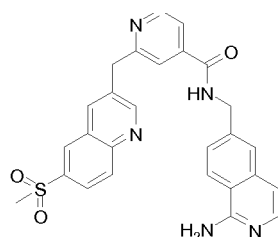
N -((1-aminoisoquinolin-6-yl)methyl)-2-((6-(methylsulfonyl)quinolin-3-yl)methyl)isonicotinamide
