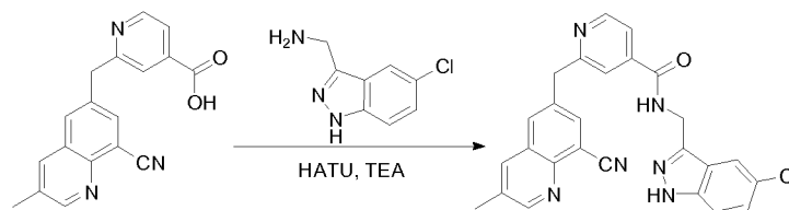
N-((5-chloro-1H-indazol-3-yl)methyl)-2-((8-cyano-3-methylquinolin-6-yl)methyl)isonicotinamide
