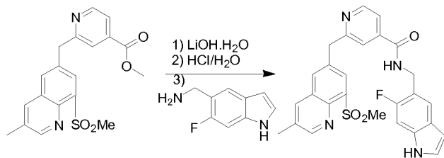
N-((6-fluoro-1H-indol-5-yl)methyl)-2-((3-methyl-8-(methylsulfonyl)quinolin-6-yl)methyl)isonicotinamide
