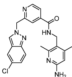
N-((6-amino-2,4-dimethylpyridin-3-yl)methyl)-2-((5-chloro-2H-indazol-2-yl)methyl)isonicotinamide
