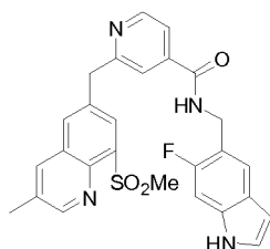
N-((6-fluoro-1H-indol-5-yl)methyl)-2-((3-methyl-8-(methylsulfonyl)quinolin-6-yl)methyl)isonicotinamide
