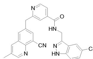
N-((5-chloro-1H-indazol-3-yl)methyl)-2-((8-cyano-3-methylquinolin-6-yl)methyl)isonicotinamide
