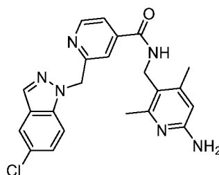
N-((6-amino-2,4-dimethylpyridin-3-yl)methyl)-2-((5-chloro-1H-indazol-1-yl)methyl)isonicotinamide
