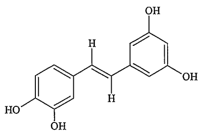
piceatannol (3,3',4',5 -tetrahydroxy stilbene)
