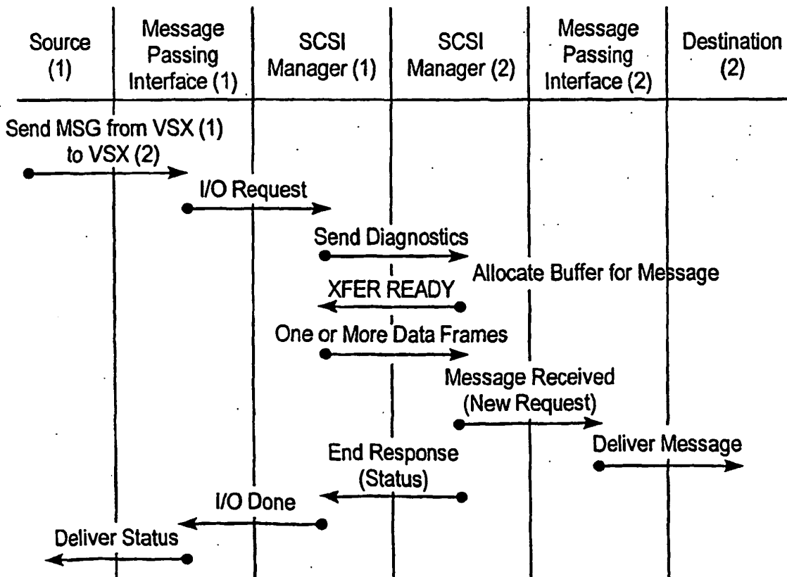
FIG. 24 VSX to VSX Message Passing
