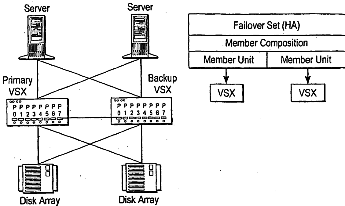
FIG. 28 2 Node HA Configuration
