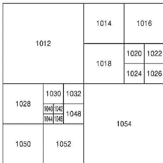
编码单元(1010)
